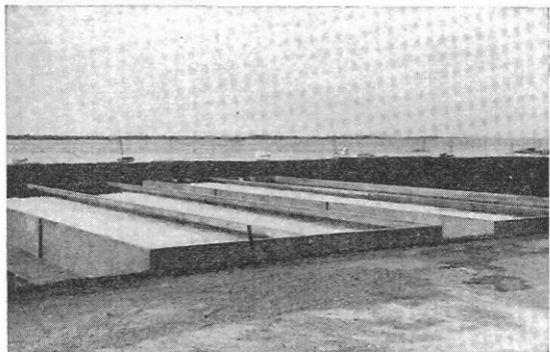
Fig. 3. — Tanques exteriores de hormigón armado donde se mantienen los peces jóvenes del Paraná hasta su transporte en camión para sembrar los ríos.
