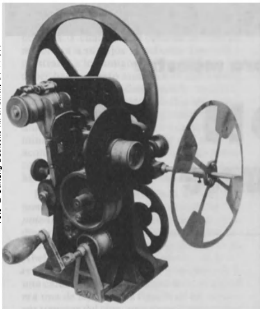
Este aparato de proyección con un mecanismo de engranaje data de 1908.
