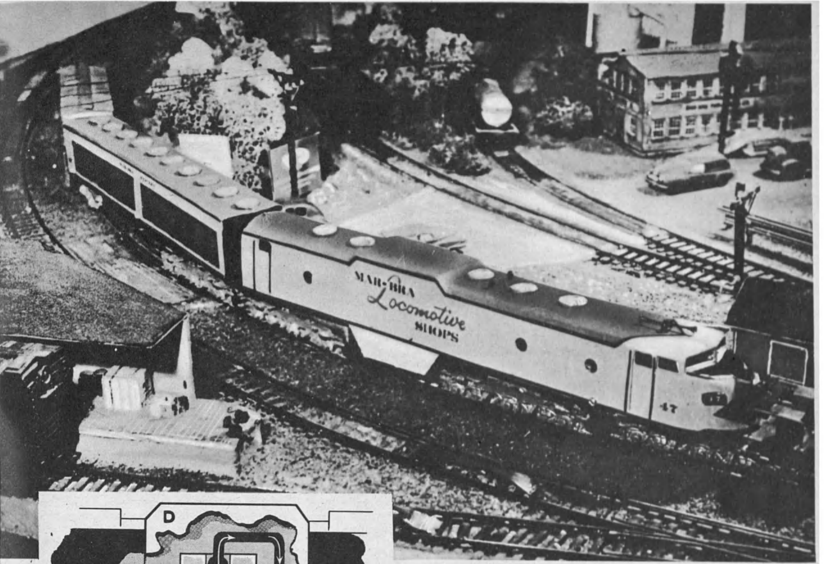
LA LOCOMOTORA MOVIDA POR ENERGIA ATOMICA no existe todavía sino en el mundo lilliputiense de los modelos construidos en la Univer- sidad de Utah, Estados Unidos de América (arriba). La parte principal de la máquina se encuentra detrás de la garita del conductor. En el corte transversal (diseño de la izquierda) se distingue el reactor nuclear (A) que contiene una solución de uranio 235. El vapor producido por este reactor debe pasar por la tubería (B) para llegar a la turbina (C) que hará funcionar cuatro generadores de electricidad. Finalmente, la electricidad producida por estos generadores pondrá en movimiento la locomotora.
