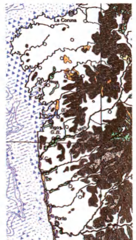
Detalle de la hoja 9 del Mapa internacional del Cuaternario de Europa (1/2.500.000).
