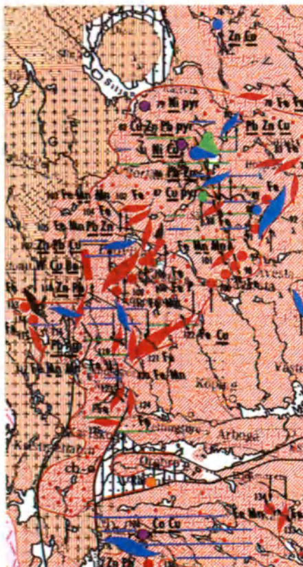
Detalle de la hoja 2 del Mapa metalogénico de Europa (1/2.500.000).
