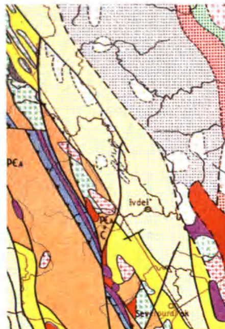
Detalle de la hoja 8 del Mapa metamórfico de Europa (1/2.500.000).
