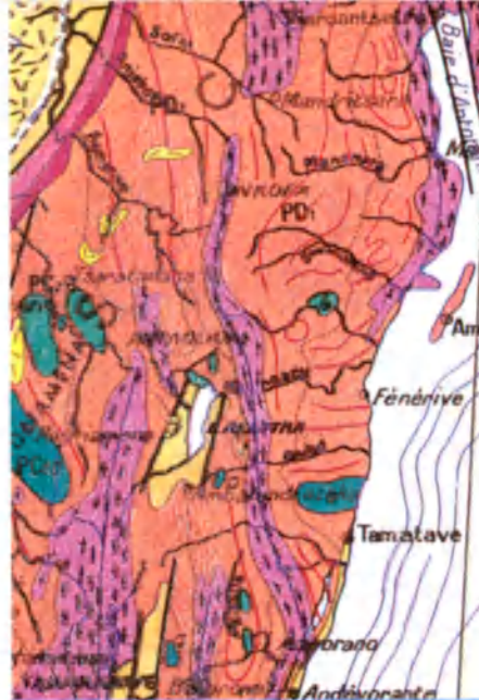
Detalle de la hoja 9 del Mapa tectónico internacional de Africa (1/5.000.000).
