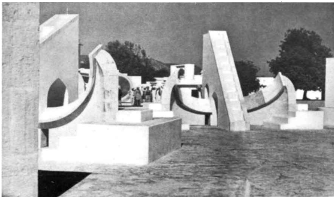
Los instrumentos de precisión del Príncipe Jai Singh, concebidos para registrar el curso de los astros, se destacan sobre el limpio cielo de la India.
