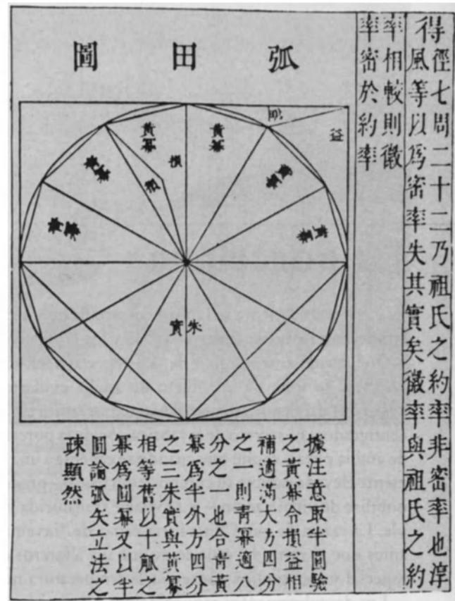
Dibujo que explica el método de aproximaciones sucesivas empleado por el matemático chino Liu Hui en el año 264 d.C. para determinar el valor del número irracional \pi .
