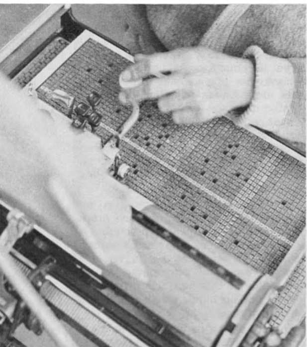
La dactilógrafa japonesa dispone de una sola tecla pero de 3 130 caracteres (o más) dispuestos en un tablero horizontal. Antes de golpear la tecla, la lleva, junto con su palanca, encima del carácter correspondiente (foto de abajo). En el papel (arriba) se imprimen los caracteres alineándose verticalmente o, si se quiere, horizontalmente.
