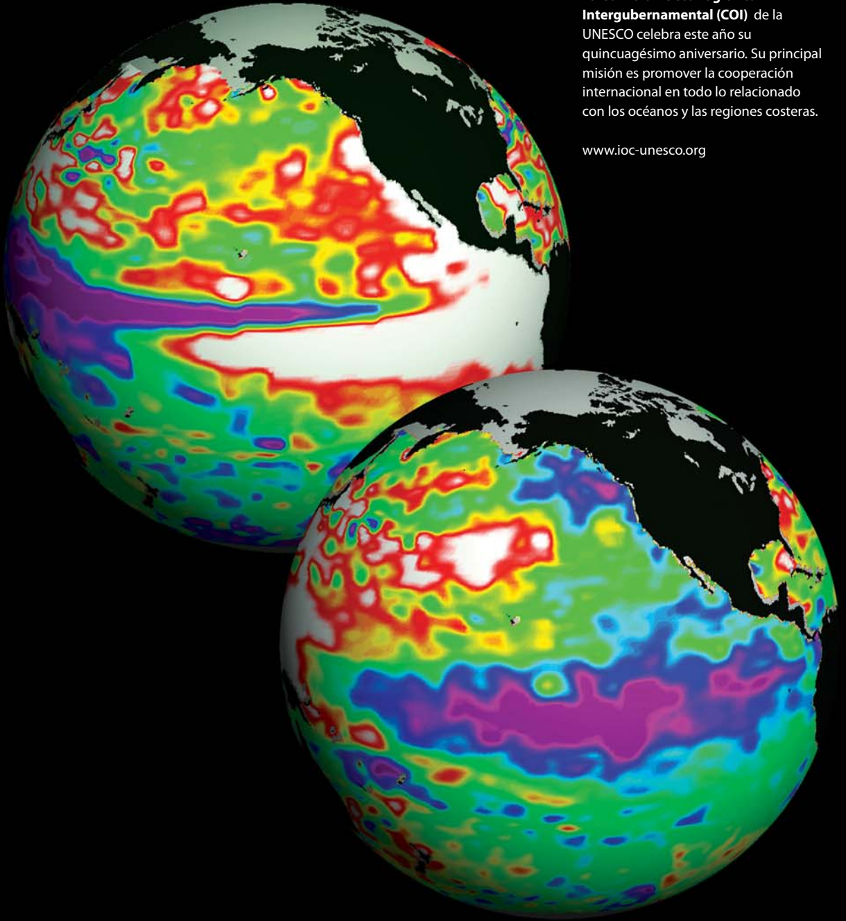
Imágenes de los fenómenos de El Niño (noviembre de 1997) y de La Niña (marzo de 1999) en el Océano Pacífico, que muestran las variaciones del nivel del mar y permiten comprender las interacciones del océano y la atmósfera susceptibles de influir en el clima.
