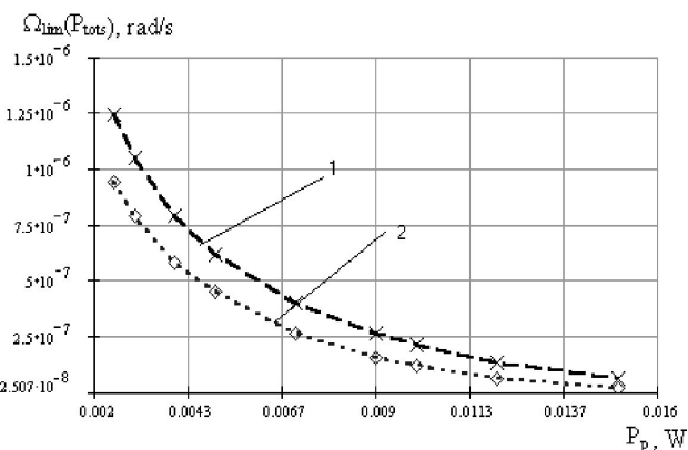
FIGURA 10. Dependencia del límite de detección \Omega_{\text{lim}}^\pm(P_{\text{tots}}^\pm) del GFO con la potencia de bombeo P_p de la FSFO, tomando en cuenta solamente el ruido de disparo, en donde: 1) dependencia \Omega_{\text{lim}}^+(P_{\text{tots}}^+) para el régimen cuando la dirección de la señal coincide con dirección de la potencia de bombeo; 2) dependencia \Omega_{\text{lim}}^-(P_{\text{tots}}^-) para el régimen cuando la dirección de la señal es contraria con la dirección de la potencia de bombeo.
