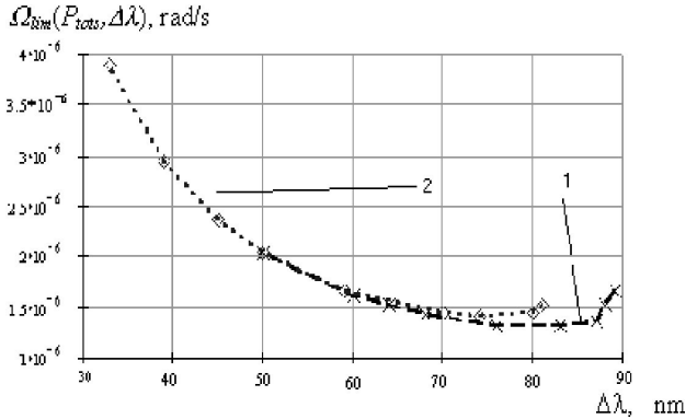
FIGURA 11. Dependencia del límite de detección \Omega_{lim}^{\pm}(P_{tots}^{\pm}, \Delta\lambda^{\pm}) del GFO con el ancho espectral \Delta\lambda^{\pm} de la señal de salida de la FSFO, tomando en cuenta las fuentes de ruido, en donde: 1) dependencia \Omega_{lim}^+(P_{tots}^+, \Delta\lambda^+) para el régimen cuando la dirección de la señal coincide con la dirección de la potencia de bombeo, 2) dependencia \Omega_{lim}^-(P_{tots}^-, \Delta\lambda^-) para el régimen cuando la dirección de la señal es contraria con la dirección de la potencia de bombeo.
