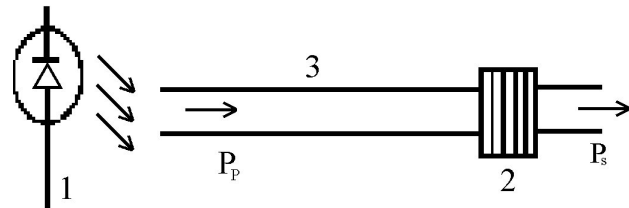
FIGURA 13. Esquema de la FSFO cuando la señal de amplificación va en dirección de la señal de bombeo en donde: 1) fuente de radiación semiconductor; 2) filtro; 3) fibra óptica activada con iones de erbio.
