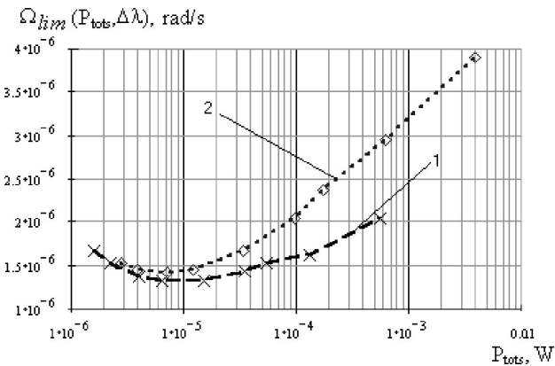
FIGURA 12. Dependencia del límite de detección \Omega_{lim}^{\pm}(P_{tots}^{\pm}, \Delta\lambda^{\pm}) del GFO con la potencia total de salida P_{tots}^{\pm} de la FSFO, tomando en cuenta las fuentes de ruido, en donde: 1) dependencia \Omega_{lim}^+(P_{tots}^+, \Delta\lambda^+) para el régimen cuando la dirección de la señal coincide con la dirección de la potencia de bombeo; 2) dependencia \Omega_{lim}^-(P_{tots}^-, \Delta\lambda^-) para el régimen cuando la dirección de la señal es contraria con la dirección de la potencia de bombeo.
