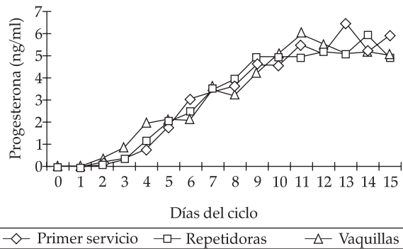
Figura 1. Concentraciones de progesterona plasmática durante los primeros 15 días posinseminación de vacas de primer servicio, vacas repetidoras y vaquillas de primer servicio. Las diferencias entre grupos no son significativas ( P > 0.05 ). Morales et al. 5
