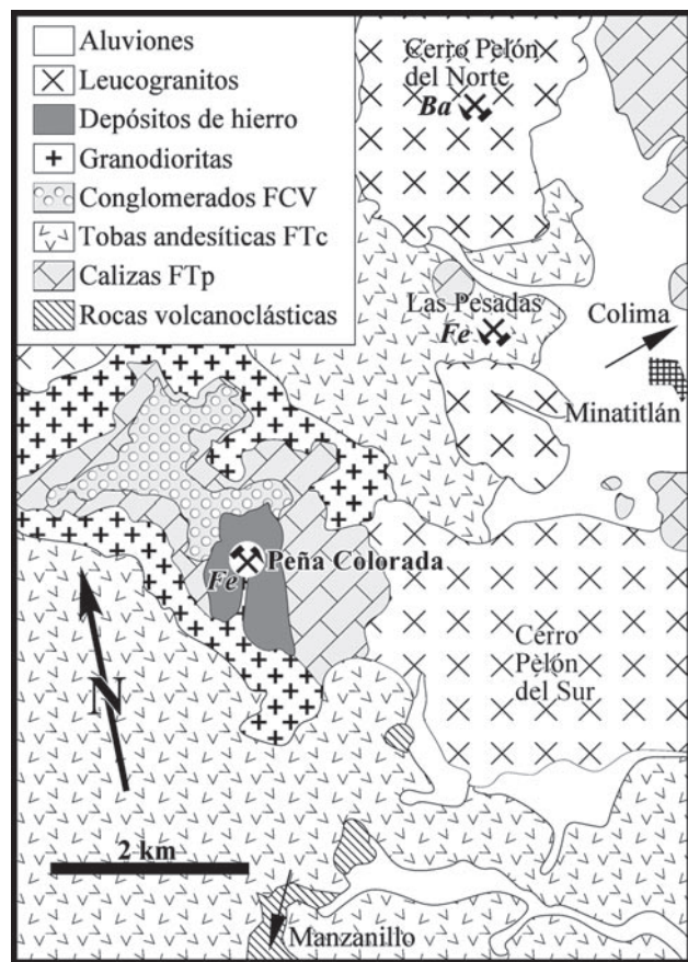
Figura 2. Mapa geológico del área de Peña Colorada (municipio de Minatitlán, Colima). Modificado del mapa geológico del Consorcio Minero Benito Juárez y de Zürcher et al. (2001).
