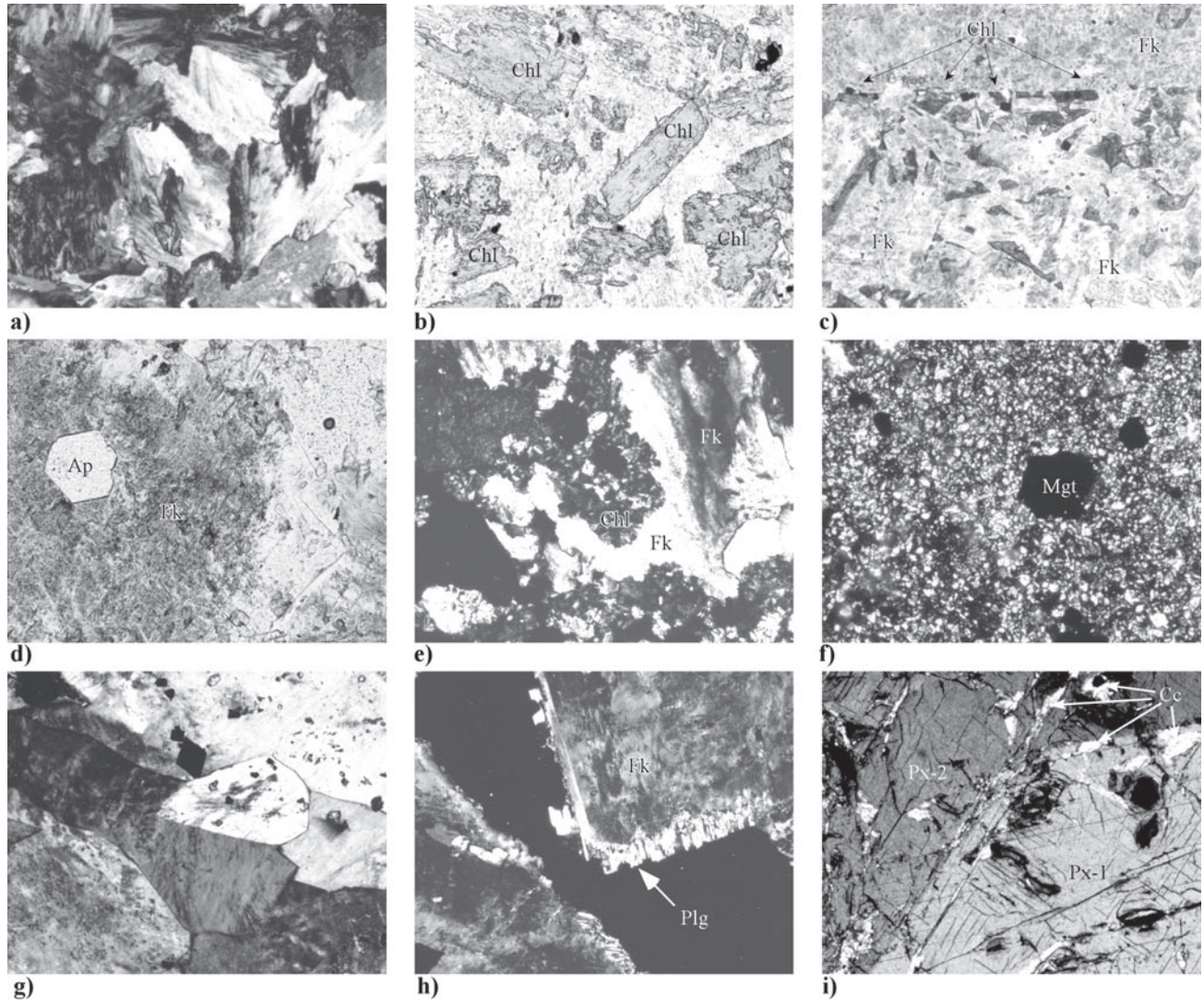
Figura 6. Microfotografías de las asociaciones minerales de los diferentes cuerpos mineralizados del depósito de Fe de Peña Colorada. “Esférulas” de feldespato potásico del cuerpo masivo superior de magnetita: a) feldespato potásico con textura “plumosa” pseudomorfizando granate (nícoles cruzados); b) y c) diversos estadios de pseudomorfosis de antiguos cristales de piroxeno englobados en feldespato potásico por clorita férrica (nícoles paralelos); d) cristales idiomórficos de apatita englobados en feldespato potásico parcialmente caolinitizado (nícoles paralelos). Nivel diseminado inferior: e) cristales de feldespato potásico de la episienita sensu lato parcialmente alterados por clorita + epidota (nícoles cruzados); f) banda rica en piroxeno microcristalino con diseminación de cristales idiomórficos de magnetita (nícoles cruzados); g) episienita sensu lato formada por cristales poiquilíticos de feldespato potásico, con inclusiones de magnetita y de apatita (nícoles cruzados); h) Cristales cristales idiomórficos de feldespato potásico creciendo en las cavidades de la episienita, parcialmente corroídos por una última generación de albita (nícoles cruzados). Brecha polymictica: i) piroxeno hedenbergítico de las “nelsonitas pobres en Ti” mostrando un fuerte zoneamiento composicional (Px-1 = zona interna; Px-2 = zona externa); estos piroxenos muestran evidencias alteración hidrotermal, con precipitación de calcita en microfracturas (nícoles cruzados). Clave: Ap = apatita, Chl = clorita, Fk = feldespato potásico, Mgt = magnetita, Plg = plagioclasa (albita), Px = piroxeno.
