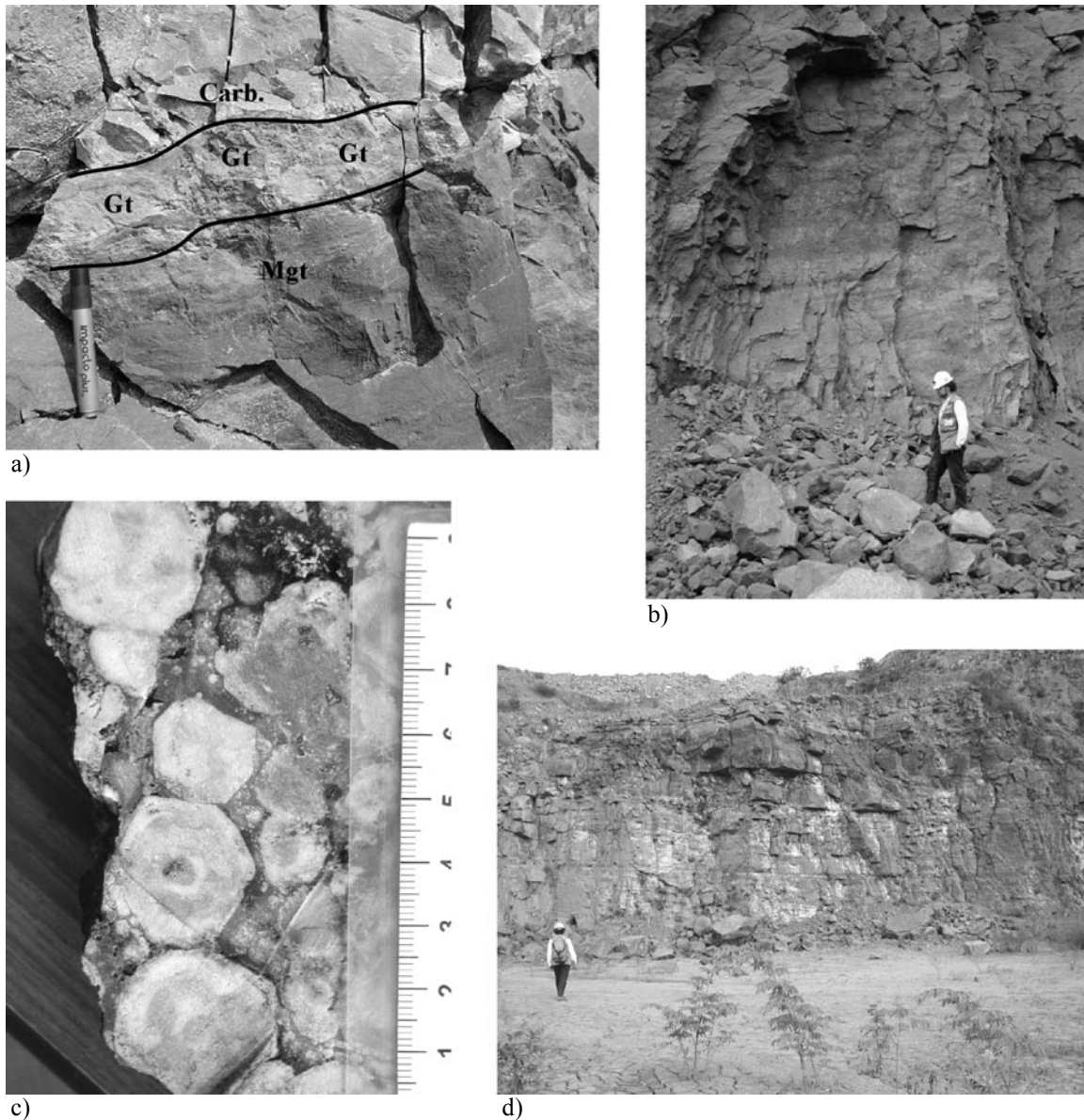
Figura 4. Fotografías del depósito de Fe de Peña Colorada. a) Detalle del contacto entre el cuerpo masivo superior de magnetita (Mgt) y las calizas sedimentarias marmorizadas (Carb) en el que se ha desarrollado un pequeño cuerpo metasomático de granate grosulárico–andradítico (Gt). b) Base del cuerpo masivo superior de magnetita en su zona de mayor grosor; el bandeamiento que se observa viene determinado por la presencia de zonas más ricas en silicatos con otras más ricas en magnetita. c) “Esférulas poliédricas” de feldespato potásico con zonación concéntrica relicta, incluidas en el cuerpo masivo superior, interpretadas como antiguos cristales de granate de composición grosularia–andradita. d) Vista general del cuerpo diseminado inferior, en que se puede apreciar el marcado bandeamiento que lo caracteriza.
