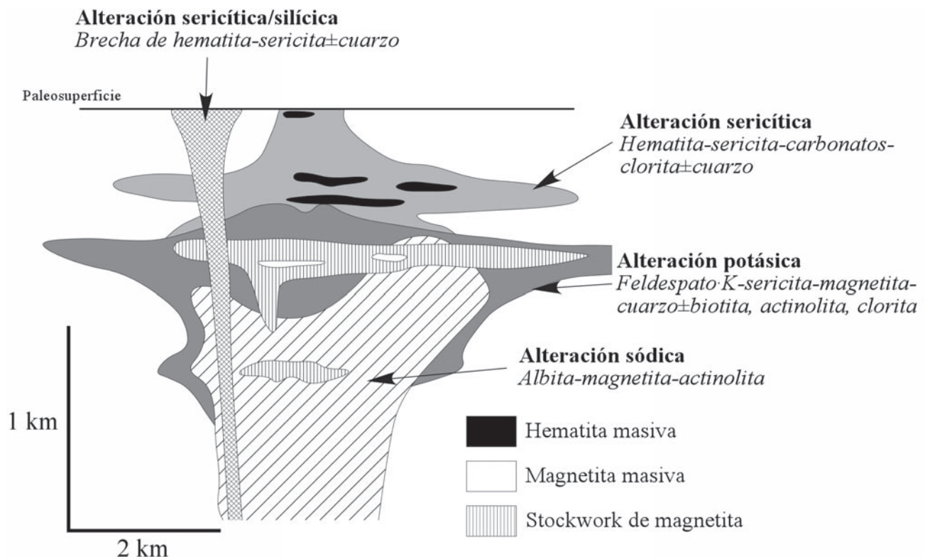
Figura 8. Sección esquemática ilustrando la disposición de los cuerpos mineralizados y de las alteraciones asociadas para los depósitos de tipo IOCG encajonados en rocas volcánicas y plutónicas proterozoicas (según Hitzman et al. , 1992).
