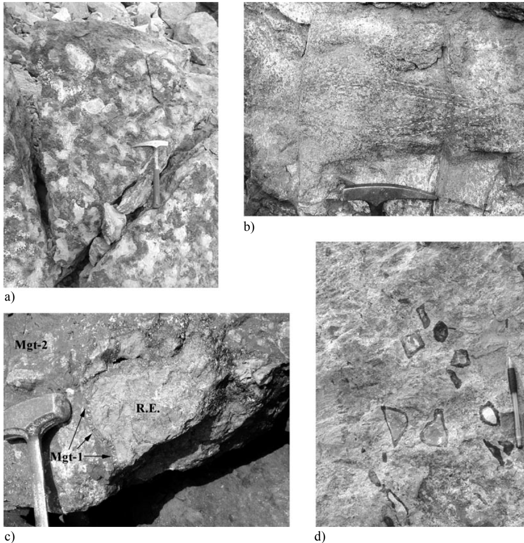
Figura 7. Fotografías del depósito de Fe de Peña Colorada. a) Cuerpo diseminado inferior; estructuras de carga desarrolladas en la interfase piroxeno–magnetita en ciclos consecutivos de pirita–magnetita–piroxeno. b) Cuerpo diseminado inferior; detalle de las bandas o “laminaciones cruzadas” (líneas blancas discontinuas) que se disponen oblicuas a la laminación principal. c) Brecha polimíctica, constituida por fragmentos de la roca encajonante (R.E.) recubiertos por una primera generación de magnetita de grano grueso (Mgt-1), y una magnetita de grano más fino (Mgt-2), actuando como matriz de la brecha. d) Base del conglomerado mineralizado donde se puede apreciar la sustitución parcial de los clastos carbonatados por una cubierta de magnetita y hematita.
