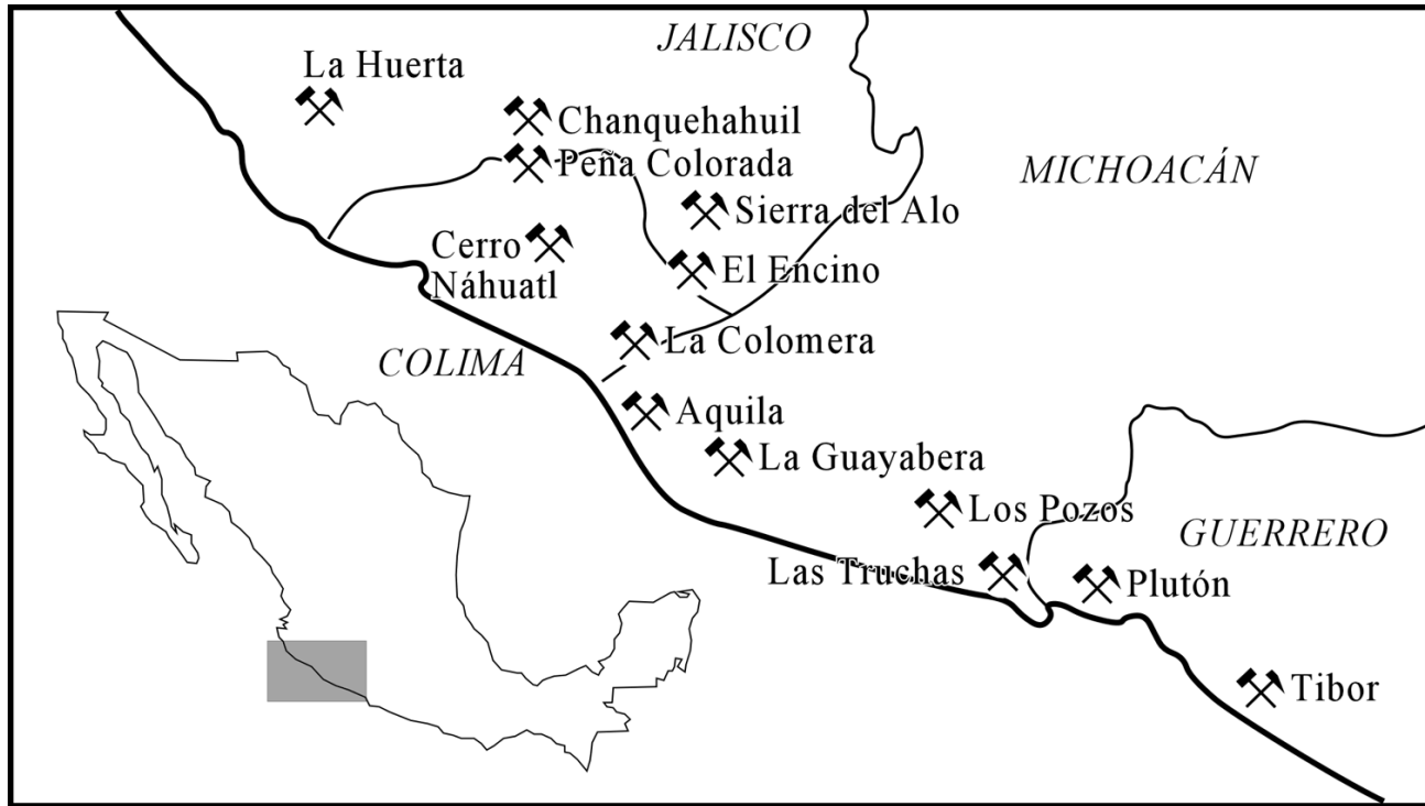
Figura 1. Mapa de localización de los principales yacimientos de Fe de la porción suroccidental de México. Modificado de Corona-Esquivel (2000).
