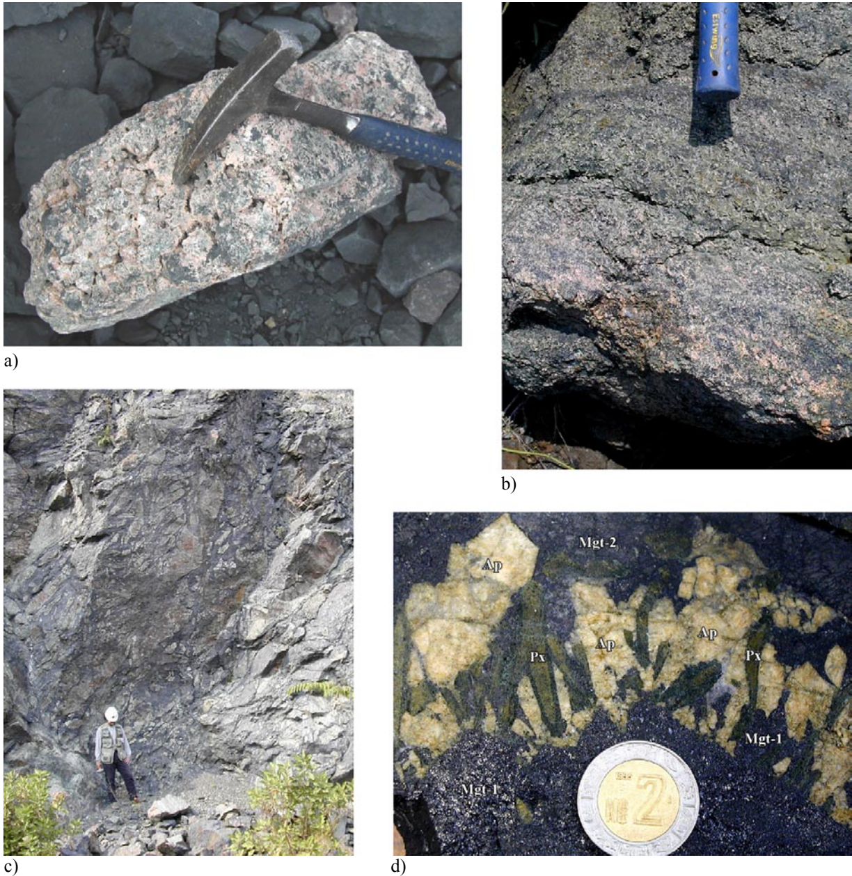
Figura 5. Fotografías del depósito de Fe de Peña Colorada. a) Cuerpo masivo superior de magnetita: acumulación de “esférulas” de feldespato potásico (sin magnetita intersticial). b) Nivel diseminado inferior: detalle de la alternancia de niveles ricos en magnetita (color negro) con niveles ricos en piroxeno (color verdoso), todos ellos con presencia de cristales poiquilíticos de feldespato potásico (color rosado) con textura isotropa. c) Parte basal de la brecha polimíctica (labores de La Chula); obsérvese como la magnetita se dispone formando la matriz de la brecha, y como los clastos de la roca encajonante pueden unirse entre sí como en un rompecabezas, sugiriendo que dicha brecha se formó mediante un mecanismo de fracturación hidráulica. d) “Nelsonita pobre en Ti”: texturas de intercrecimiento apatita–piroxeno nucleándose sobre megacristales de magnetita temprana (Mgt-1), todo ello cementado por una magnetita tardía (Mgt-2) de grano más fino. Clave: Ap = apatita, Mgt = magnetita, Px = piroxeno.
