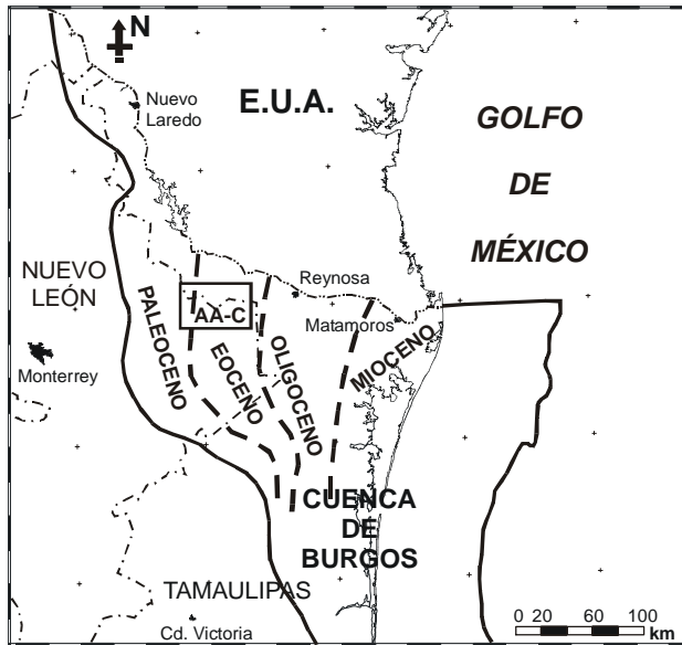
Figura 2. Franjas geológicas de la Cuenca de Burgos (AA-C: área Arcabuz–Culebra). Modificada de Echánove (1986).
