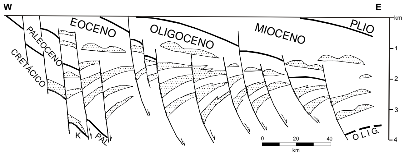
Figura 3. Sección esquemática transversal de la Cuenca de Burgos mostrando su arquitectura regional (modificada de González y Holguín, 1992).
