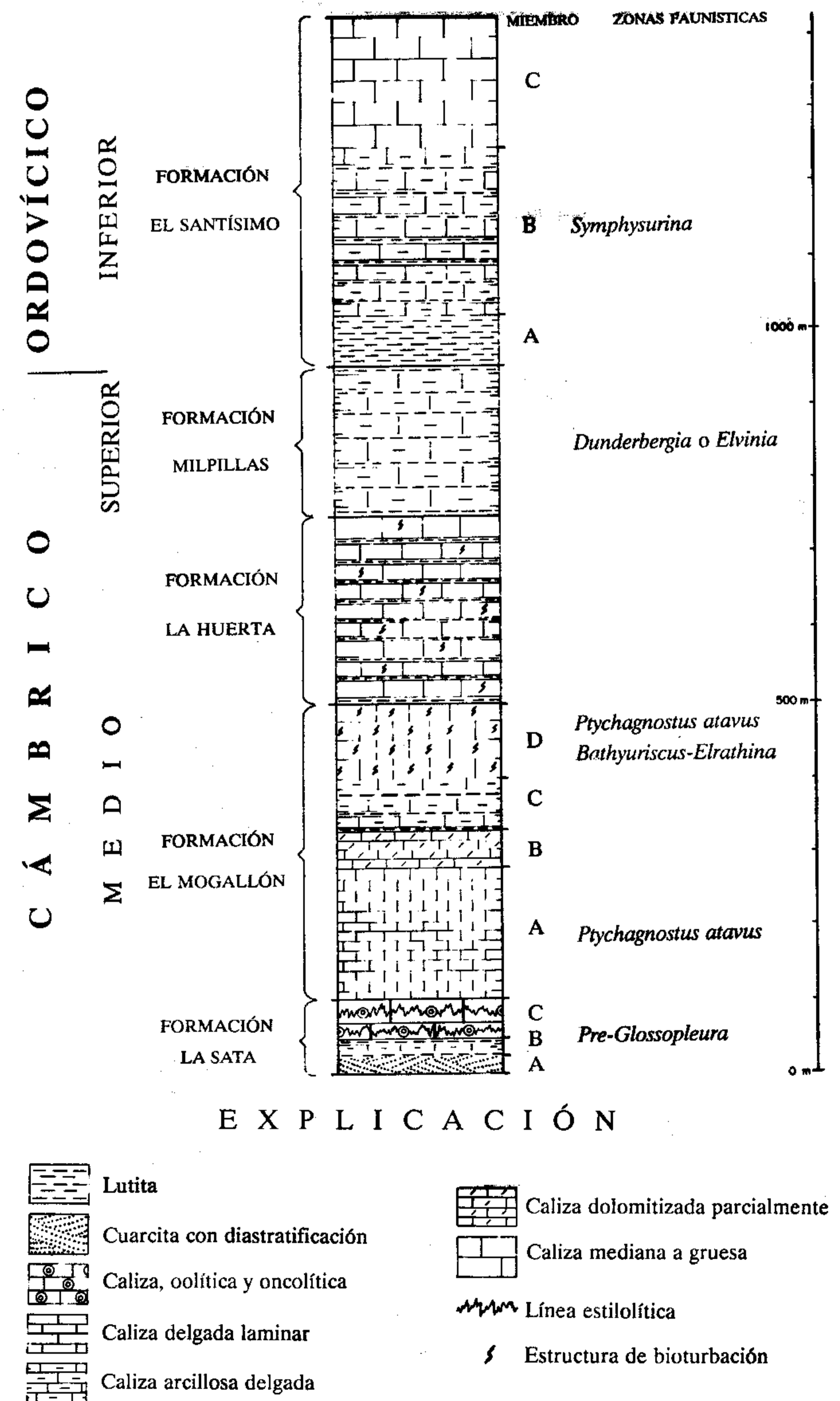
Figura 2.- Columna estratigráfica del Cámbrico y Ordovícico de la región de Arivechi, en Sonora centrooriental.
