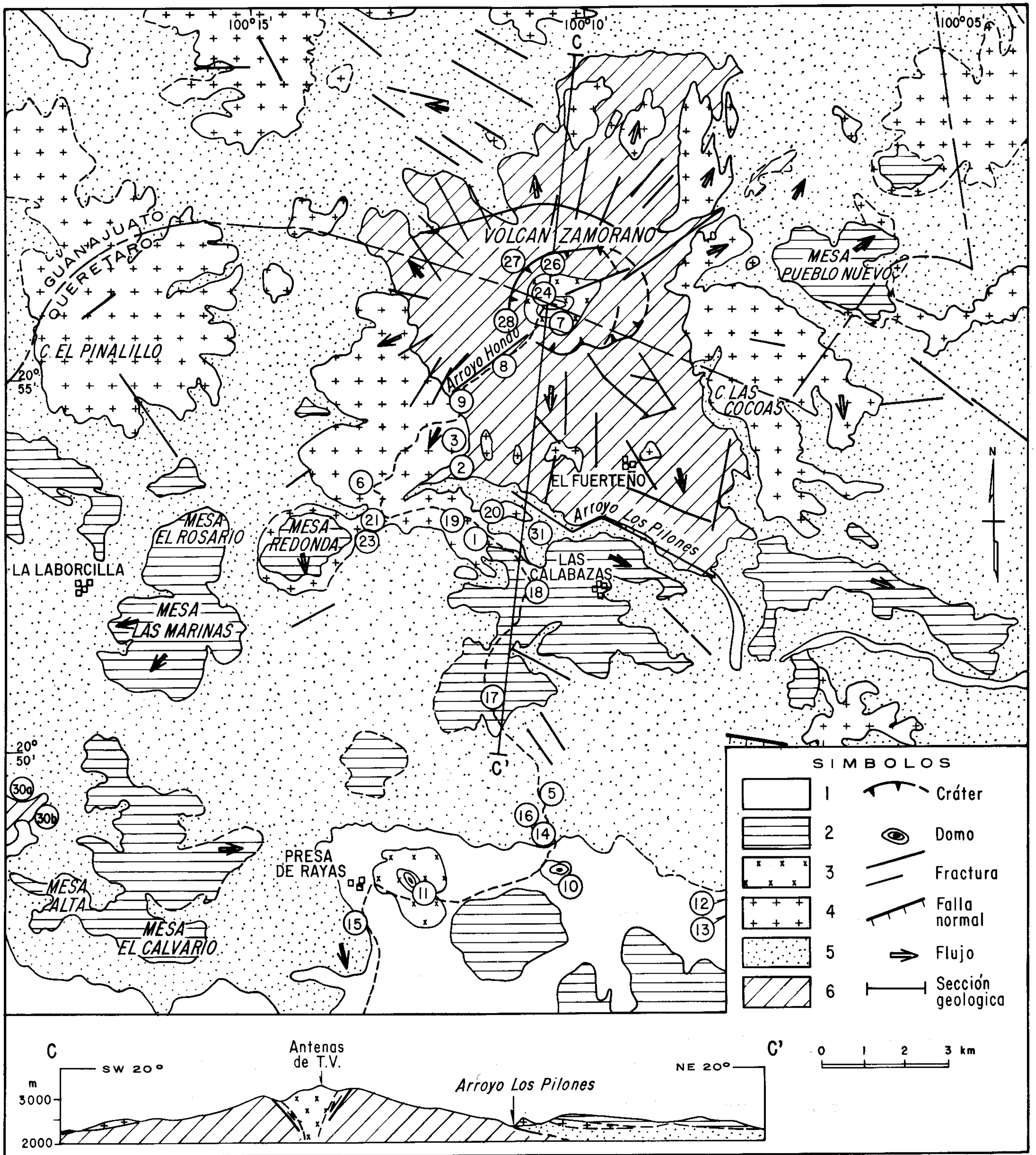
Figura 3.- Mapa geológico del área que comprende el volcán Zamorano (modificado de Carrasco-Núñez, 1988). Símbolos: 1 = aluvión; 2 = andesita Mesa Redonda; 3 = dacita del domo central; ignimbrita Zamorano 4 = unidad superior, 5 = unidad inferior; 6 = andesita Arroyo Hondo. Los números encerrados por un círculo corresponden a las muestras empleadas en este artículo; para fines prácticos se eliminó el prefijo "ZA".
