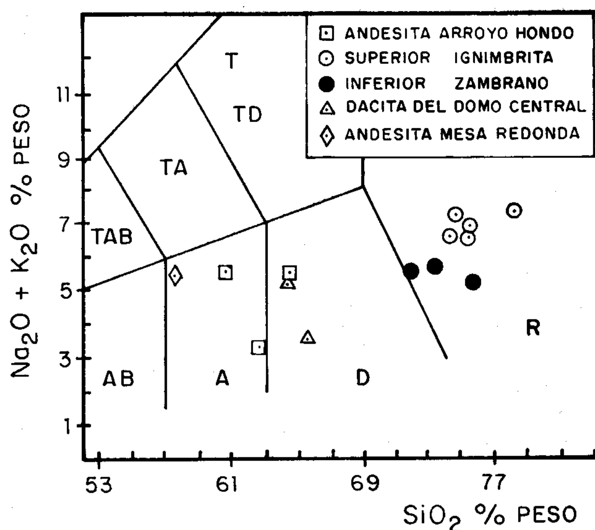
Figura 6.- Diagrama TAS ( Total Alkali-Silica ) propuesto por Le Bas y colaboradores (1986) como una clasificación geoquímica de las rocas ígneas. Clave: TAB = traquiandesita basáltica; TA = traquiandesita; TD = traquidacita; T = traquita; AB = andesita basáltica; A = andesita; D = dacita y R = riolita.
