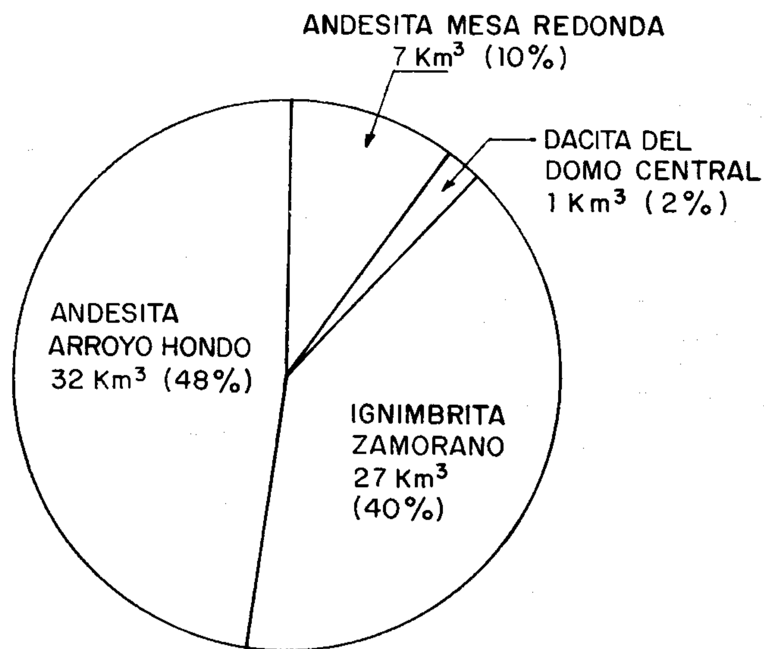
Figura 4.- Porcentaje del volumen de las unidades de roca que componen el volcán Zamorano.
