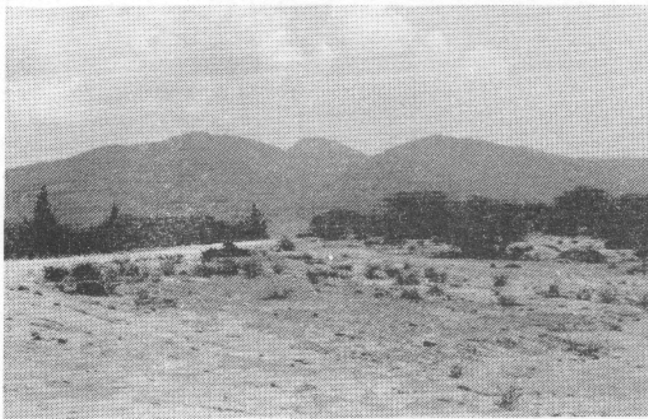
Figura 2.- Perfil característico del volcán Zamorano con un domo ocupando el centro del cráter. En primer plano, se observa los derrames ignimbríticos asociados al volcán.
