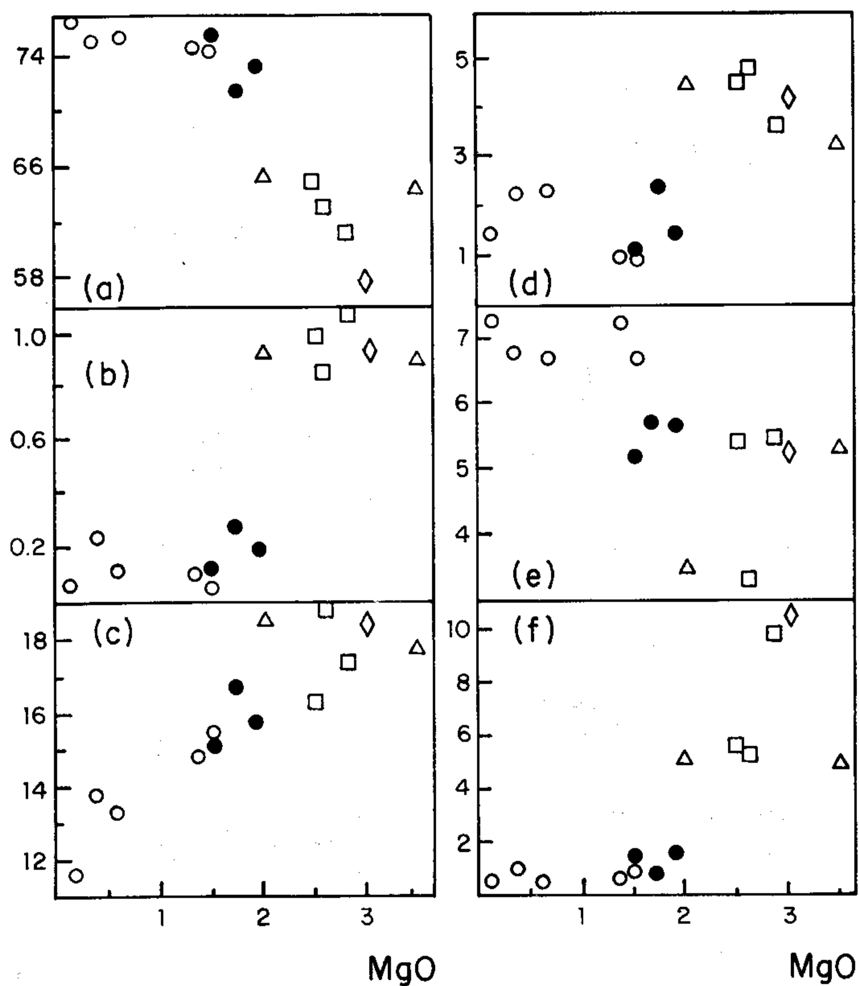
Figura 7. Diagramas de variación de óxidos vs. MgO. Símbolos iguales a los utilizados en la Figura 6. (a) SiO 2 , (b) TiO 2 , (c) Al 2 O 3 , (d) FeO total (e) Na 2 O 4 K 2 O, (f) CaO.
