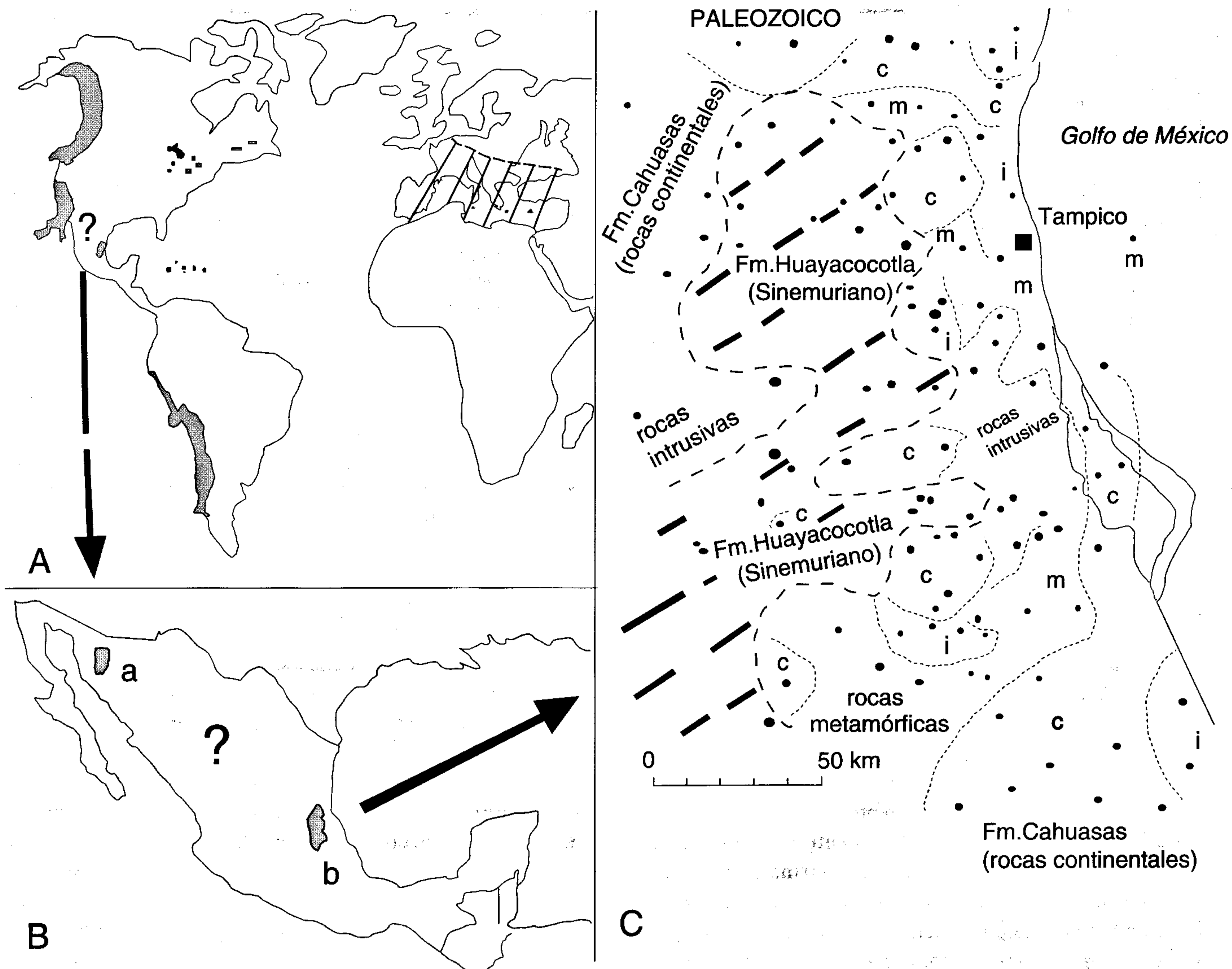
Figura 2. A, El Jurásico Inferior de la Provincia del Pacífico Oriental y del Tethys; B, dos áreas de sedimentación marina del Sinemuriano en México: Sonora (a) y Sierra Madre Oriental-subsuelo del este de México (b); C, distribución de la Formación Huayacocotla (Sinemuriano), en el subsuelo del este de México, según material de pozos petroleros; configura una paleobahía paralela a la actual línea de costa del Golfo de México y está limitada por rocas de diferente origen (c, continentales; m, metamórficas; i, intrusivas).
