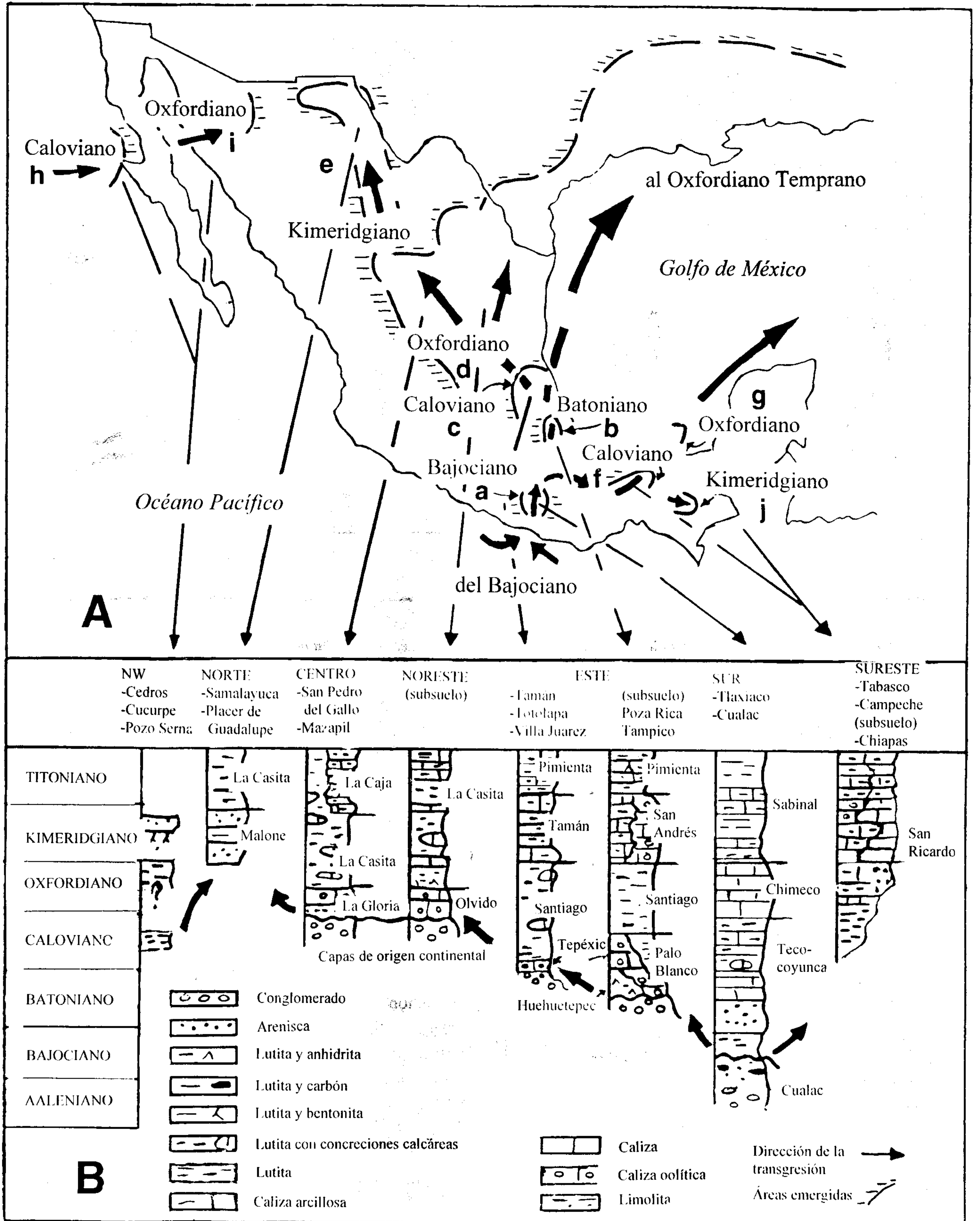
Figura 4. A, Eventos transgresivos del Jurásico Medio y Tardío en México, cuyo origen fue el ancestral Océano Pacífico, durante el Bajociano en el sur y el Caloviano en el noroeste del país. Dirección de las transgresiones hacia el norte y la actual área del Golfo de México, en el Kimeridgiano temprano y Oxfordiano temprano, respectivamente; B, correlación estratigráfica de rocas de esas edades. Eventos transgresivos (A): Oaxaca, a; Metlatoyuca, b; Huehuetla, c; Mazapil, d; Samalayuca, e; Boquiapan, f; Balam, g; Cedro, h; Cucurpe, i; Chiapas, j.
