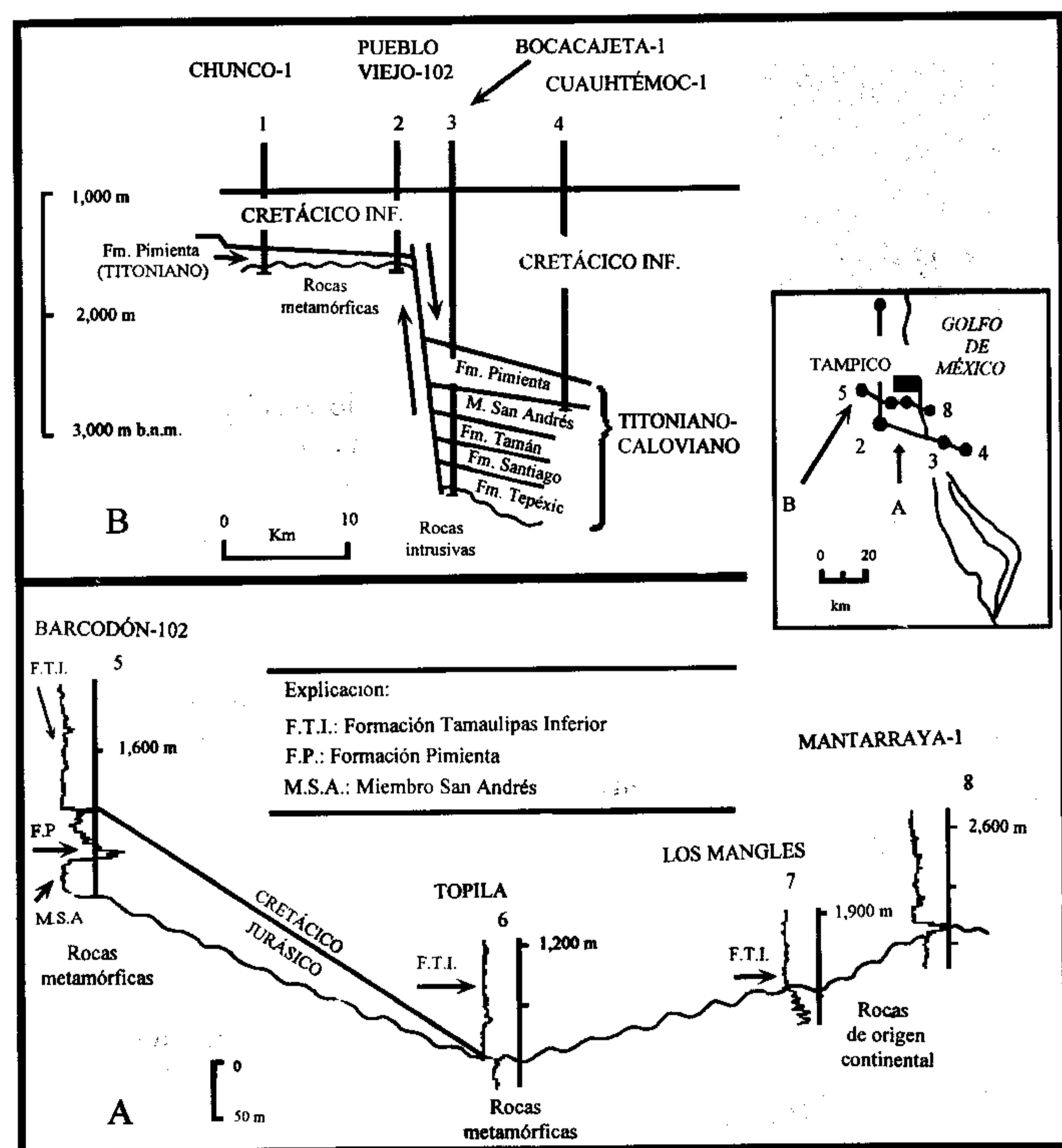
Figura 11. A, Sección estratigráfica elaborada con registros de rayos gama, de pozos de la región de Tampico, este de México. El ciclo sedimentario se inicia en la cima del Jurásico o en la base del Cretácico, sobre rocas de origen metamórfico (pozos Barcodón 102 y Topila 105) o continental (pozos Los Mangles 1 y Mantarraya 1). Horizonte de referencia: cima del Jurásico y contacto de la discordancia (Cantú-Chapa, 1989). B, Sección estratigráfico-estructural de pozos de la misma región, que muestra dos etapas del ciclo sedimentario neojurásico (pozos Chunco 1 y Pueblo Viejo 102) o mesojurásico (pozo Bocacajeta 1), depositado sobre diferentes rocas del Complejo Basal.
