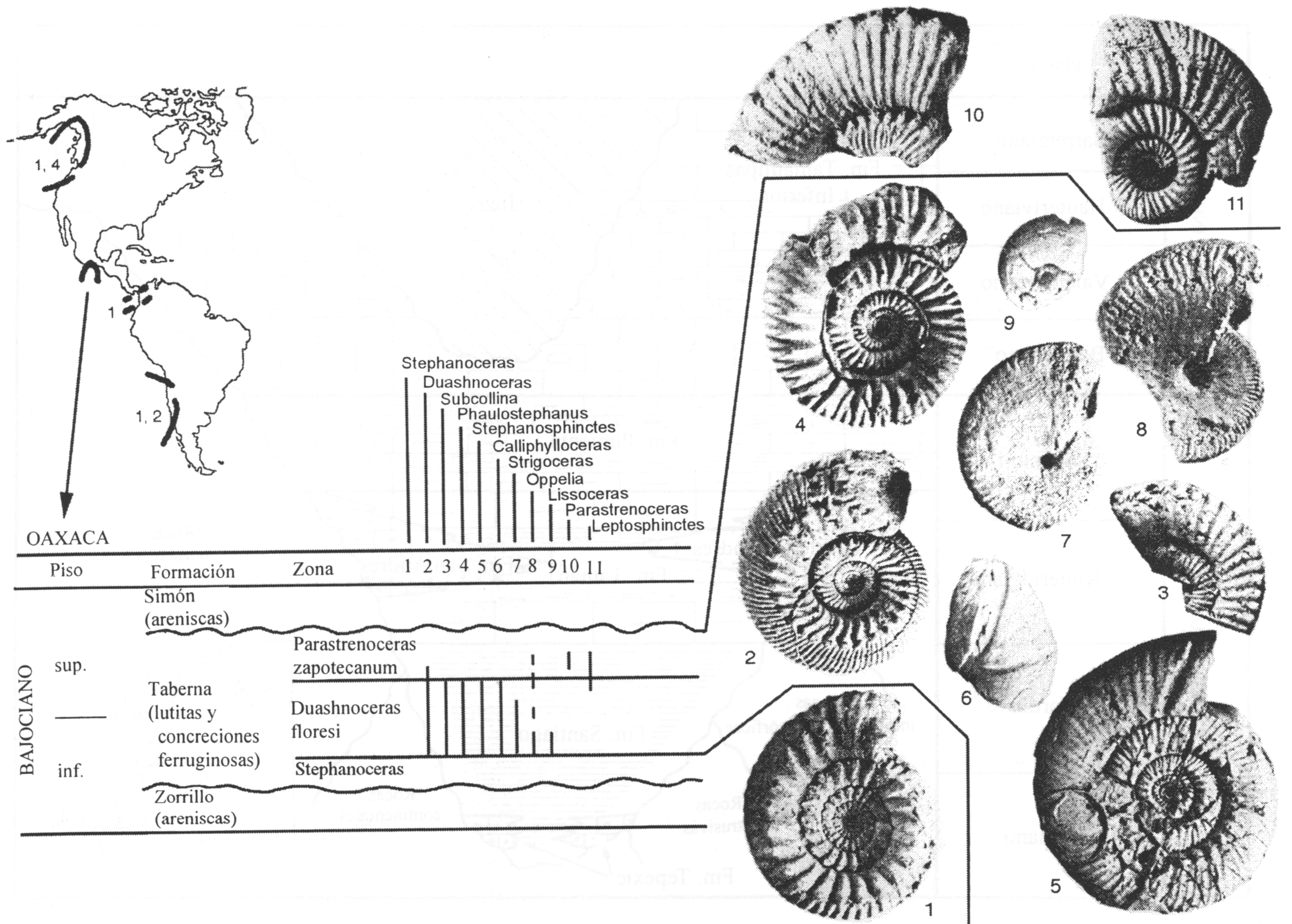
Figura 7. Bioestratigrafía y relaciones paleogeográficas de los amonites de la Formación Taberna (Bajociano) en Oaxaca, con provincias de la margen occidental del continente americano; ilustraciones de fósiles según Sandoval y Westermann (1986).
