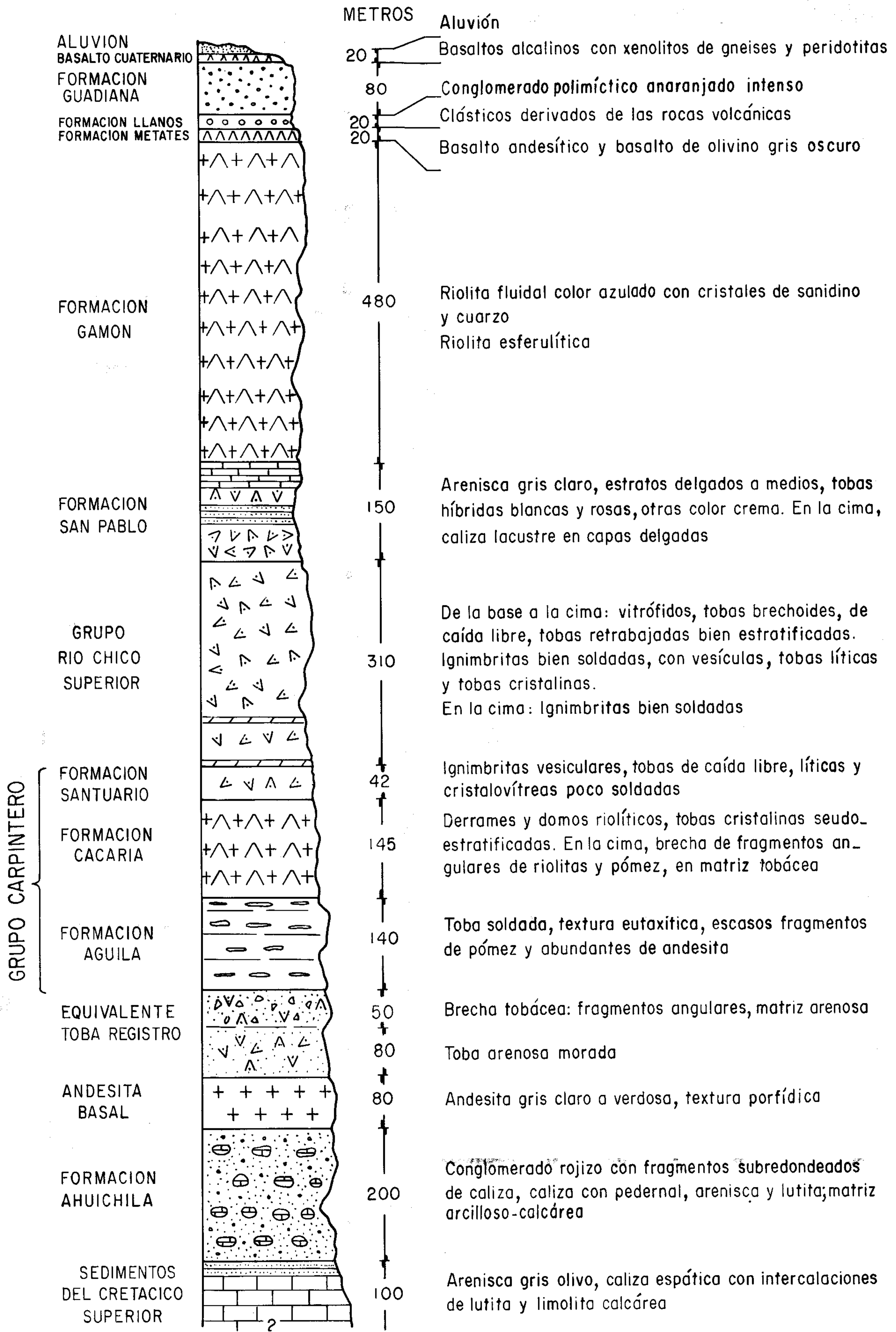
Figura 3.- Columna estratigráfica generalizada del área de las Sierras de Cacara, San Lucas, La Silla y Gamón.
