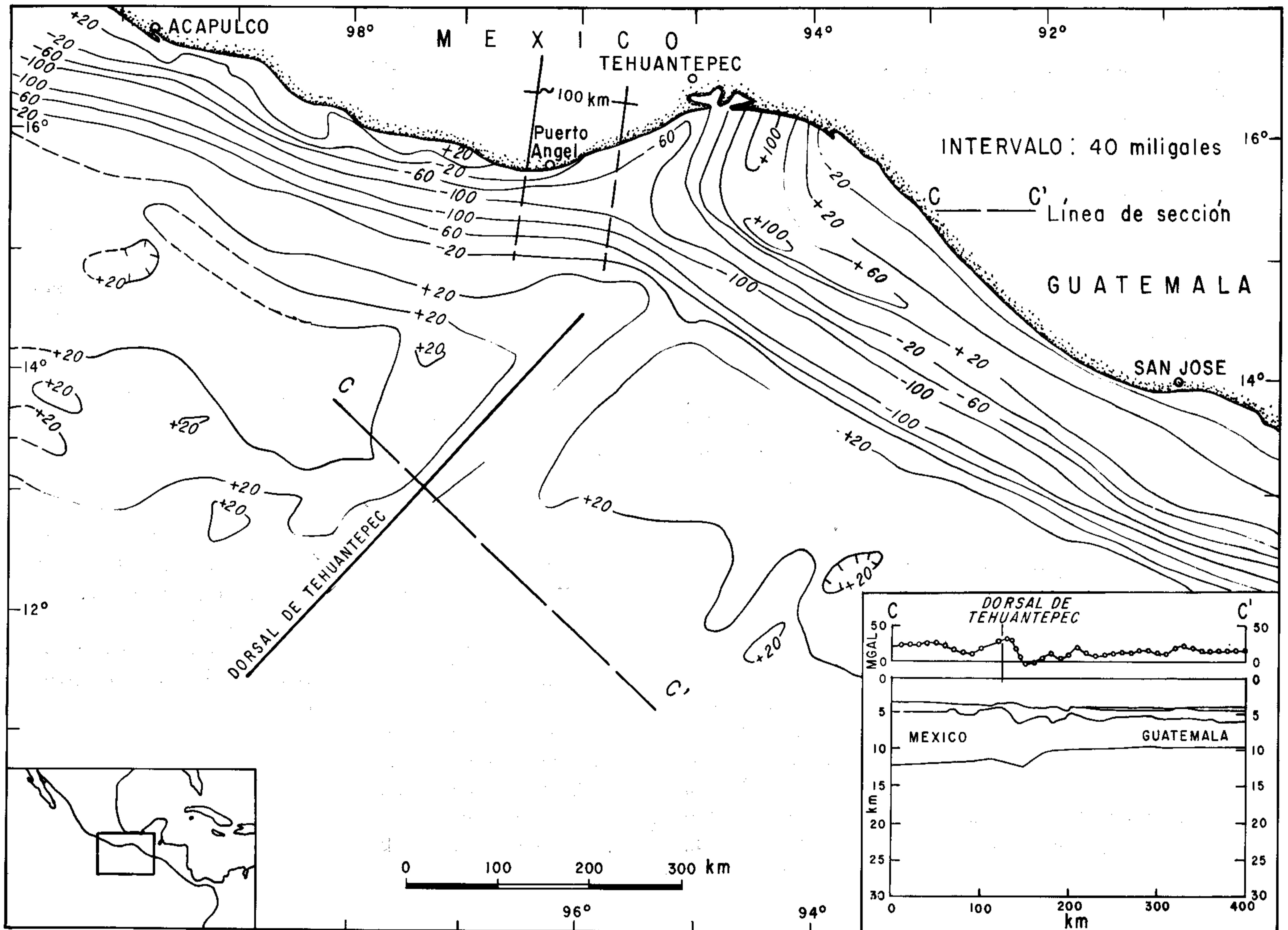
Figura 2.- Mapa de anomalías de gravedad de aire libre de la margen continental del sur de México y Guatemala, y sección cortical de la placa de Cocos, perpendicular a la dorsal de Tehuantepec (tomados de Couch y Woodcock, 1981). Se observa el cambio de orientación de la trinchera en un segmento de aproximadamente 100 km, al sur de Puerto Ángel.
