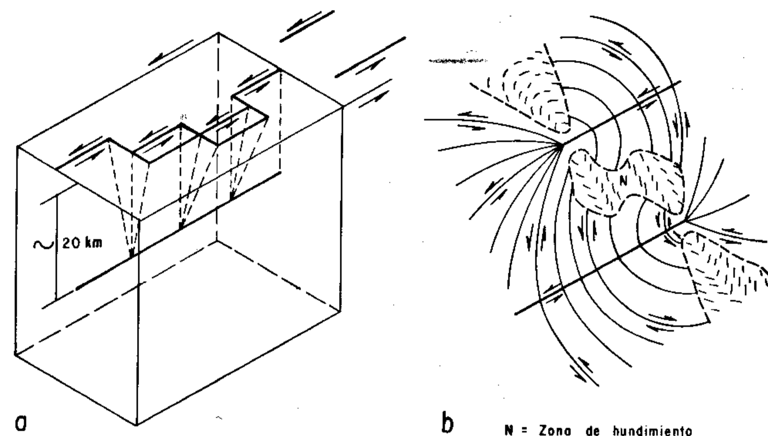
Figura 7.- (a) Bloque esquemático de un sistema transpresivo izquierdo, donde se muestra la unión de diferentes segmentos a una profundidad de aproximadamente 20 km, según el modelo sísmico de Segall y Pollard (1980). (b) Modelo de Rodgers (1980) sobre la potencial expresión superficial de un patrón de fallas, cuando las fallas principales tienen una separación de 20 km y los frentes de éstas se traslapan 10 km.
