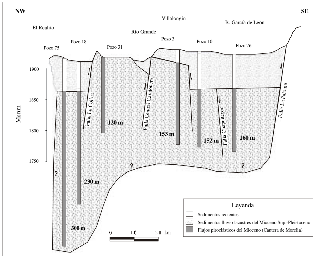
Figura 6. Perfil norte-sur de la Ciudad de Morelia, donde con la información derivada de la perforación de los pozos para agua se ha configurado el comportamiento de las ignimbritas del Mioceno (Cantera de Morelia). Se observa con mucha claridad que fallas como La Paloma y Central Camionera tienen una gran expresión en el subsuelo.
