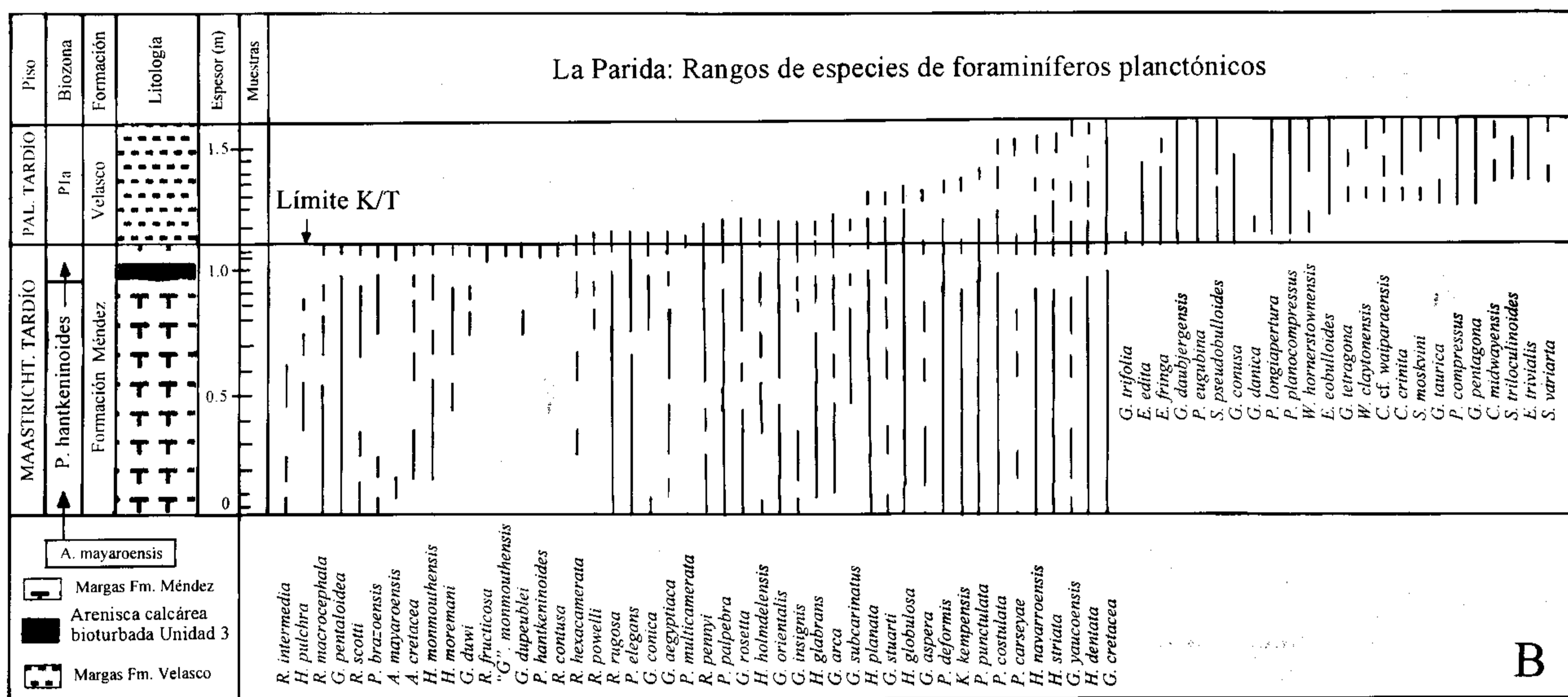
Figura 3. Sucesión de especies de foraminiferos planctónicos. A, área El Mulato; B, área La Parida.
