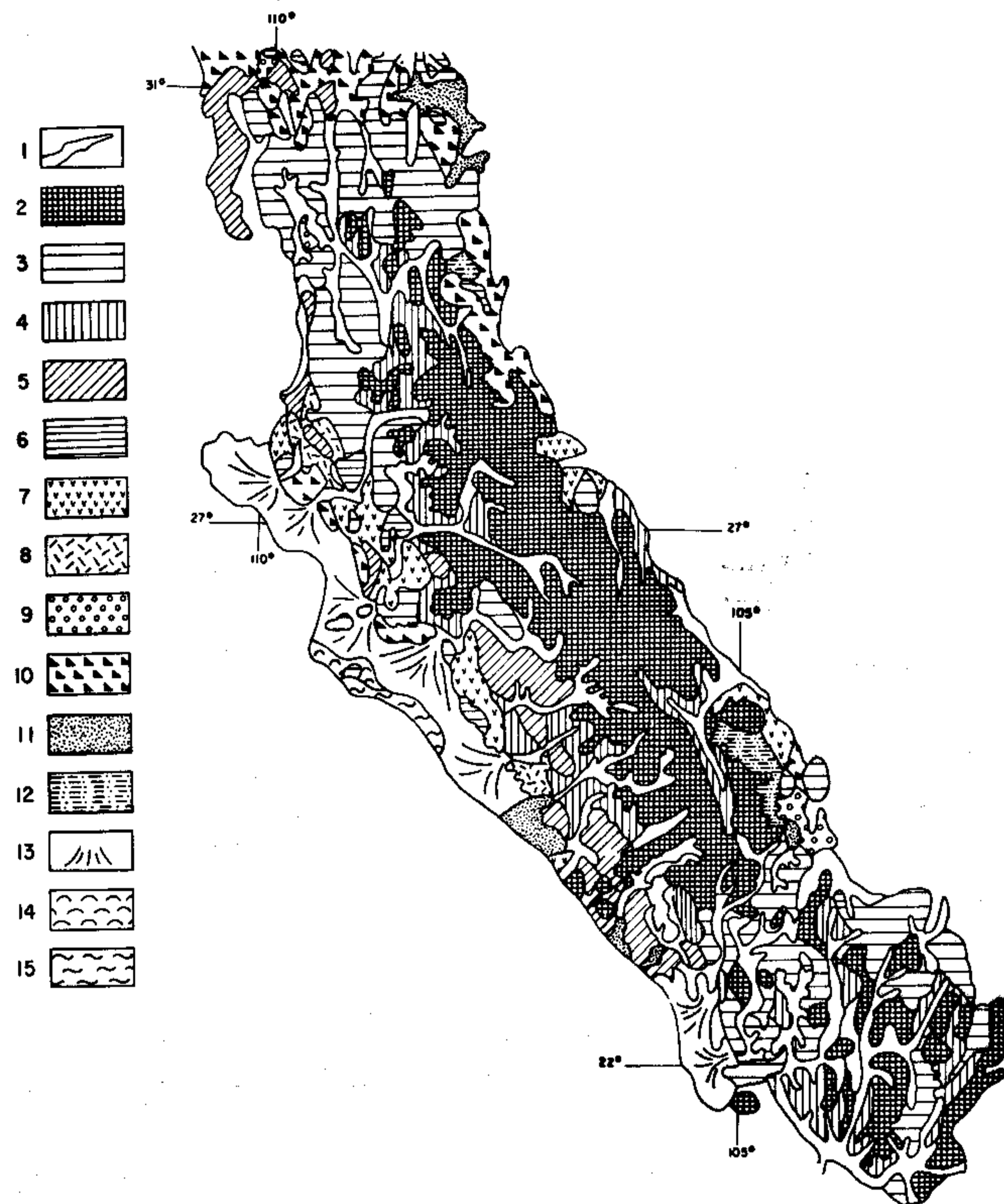
Figura 6.- Formas del relieve de la Sierra Madre Occidental (Lugo-Hubp y Córdoba-Fernández de Arteaga, 1990). 1, Valles erosivos (Q); 2, Mesas de riolita (Oligoceno-Plioceno); 3, Elevaciones montañosas de riolitas; 4, Ladera escarpada (margen exterior) de la Sierra Madre Occidental; 5, Elevaciones plegadas o de bloque con cubierta volcánica del Neógeno-Cuaternario; 6, Elevaciones menores de riolitas (Oligoceno-Plioceno); 7, Lomeríos volcánicos (N-Q); 8, Lomeríos de rocas intrusivas y metamórficas; 9, Campos volcánicos cuaternarios (conos monogenéticos, piroclastos y lavas); 10, Superficies de piedemonte de acumulación proluvial (Q); 11, Planicies de acumulación fluvial (Q); 12, Planicies de acumulación fluvio-lacustre (Q); 13, Planicies de acumulación deltaica (13); 14, Planicies de acumulación marina-eólica (Q); 15, Planicies de acumulación marina (Q).
