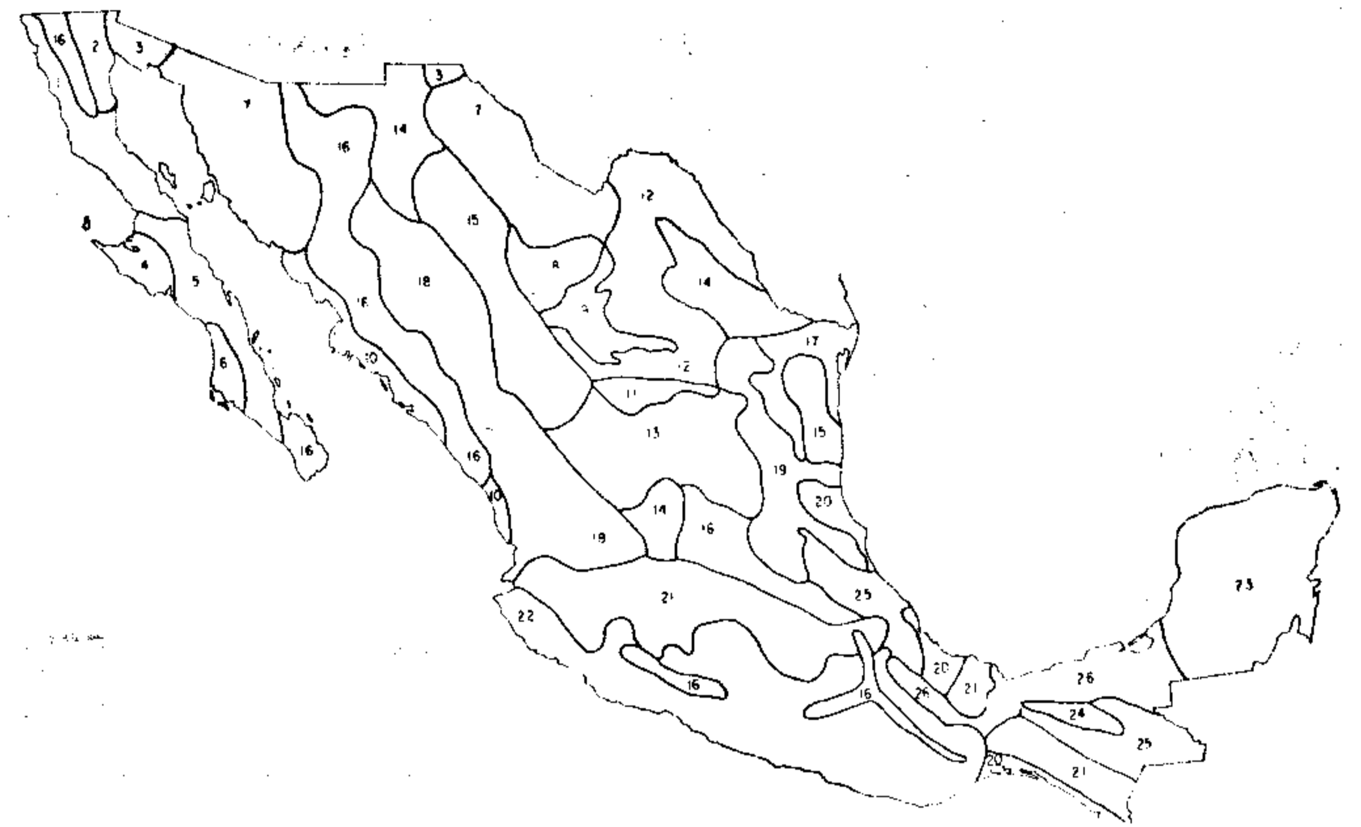
Figura 4.- Mapa de regionalización de los procesos exógenos actuales en la República Mexicana. (Elaborado con base en García-Amaro, 1990; Lugo-Hubp, 1990; Lugo-Hubp y Córdoba-Fernández de Arteaga, 1990a, 1990b). Regiones muy áridas: 1, Erosión fluvial; 2, Erosión fluvial, procesos gravitacionales y acumulación del piedemonte (proluvial); 3, Acumulación eólica; 4, Erosión y acumulación eólica; 5, Erosión remontante; 6, Acumulación proluvial; 7, Erosión (procesos gravitacionales) y acumulación proluvial; 8, Erosión y acumulación fluvial; 9, Acumulación proluvial y eólica; 10, Acumulación fluvial deltaica. Regiones áridas: 11, Acumulación fluvial y proluvial; 12, Erosión fluvial; 13, Erosión y acumulación proluvial. Regiones subáridas: 14, Erosión y acumulación proluvial; 15, Erosión y acumulación fluviales; 16, Erosión fluvial; 17, Acumulación fluvial. Regiones subhúmedas: 18, Erosión fluvial vertical y remontante; 19, Erosión fluvial y carso; 20, Acumulación fluvial; 21, Erosión fluvial, acumulación fluvial, lacustre y proluvial; 22, Erosión fluvial y carso (en localidades pequeñas); 23, Carso. Regiones húmedas: 24, Erosión fluvial; 25, Carso; 26, Acumulación fluvial y deltaica.
