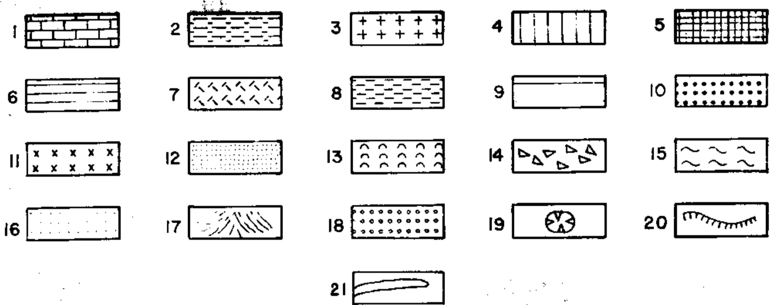
Figura 10.- Formas del relieve en el sudeste de México (Lugo-Hubp y Córdova-Fernández de Arteaga, 1990). 1, Montañas de rocas plegadas (mesozoico-terciarias); 2, Altiplanicies estructurales de rocas sedimentarias mesozoicas; 3, Montañas de bloque de rocas intrusivas mesozoicas; 4, Elevaciones de acumulación riolítica (Neógeno ?); 5, Elevaciones montañosas de bloque o plegadas con cubierta volcánica neogénica; 6, Elevaciones montañosas con estructura monoclinial (rocas mesozoico-cenozoicas); 7, Lomeríos de rocas intrusivas mesozoicas; 8, Lomeríos de rocas sedimentarias mesozoicas; 9, Lomeríos de rocas sedimentarias cenozoicas; 10, Campo volcánico cuaternario; 11, Planicie de acumulación volcánica; 12, Planicie de acumulación fluvial; 13, Planicie de acumulación marino-eólica; 14, Superficie de acumulación de piedemonte; 15, Planicie de acumulación lacustre; 16, Planicie de acumulación marina; 17, Planicie deltaica; 18, Piedemonte volcánico (tefra y lava); 19, Volcanes compuestos (potencialmente activos); 20, Escarpes principales; 21, Valles erosivos.
