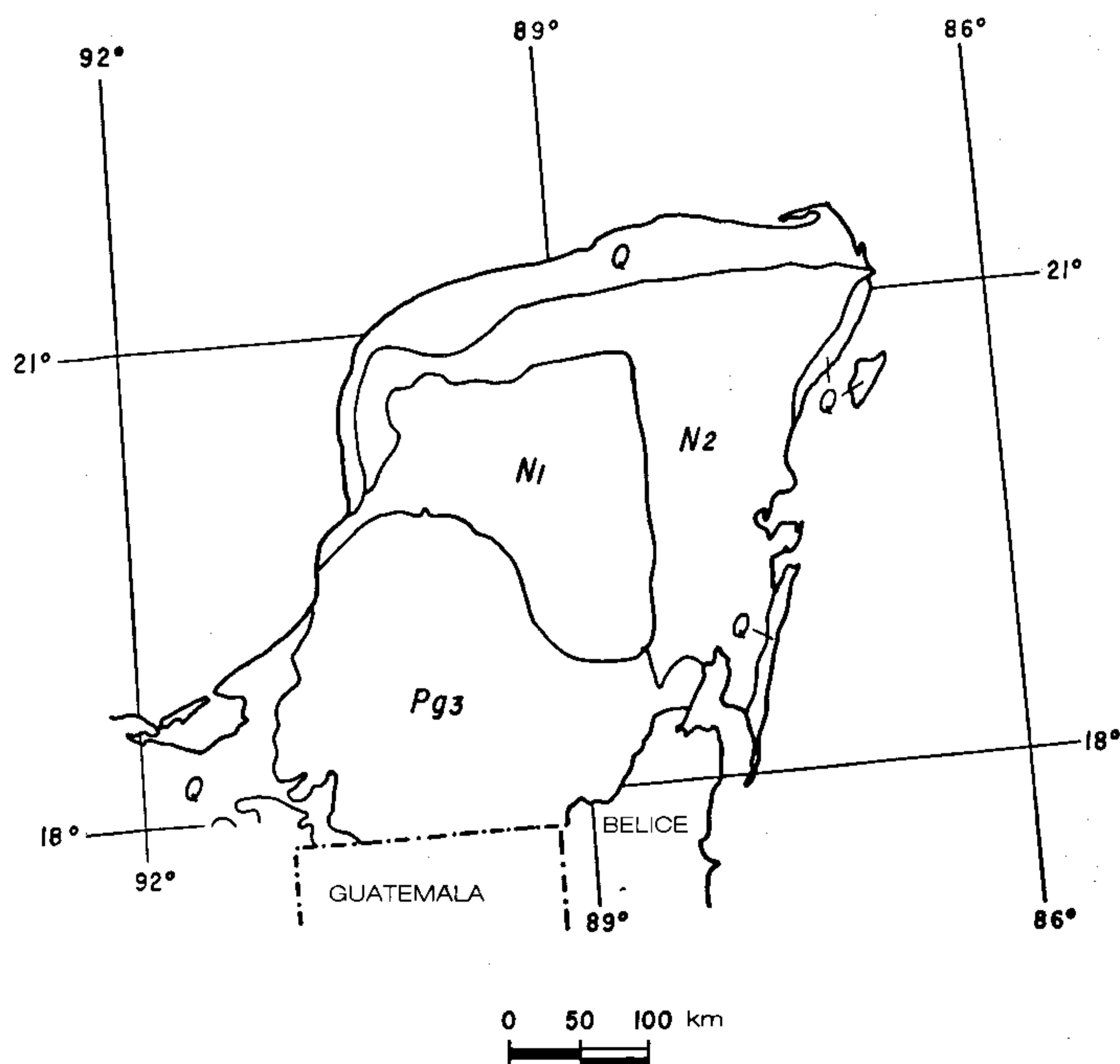
Figura 2.- Geología de la península de Yucatán (tomado de López-Ramos, 1975). Q—Cuaternario; N2—Neógeno superior: Plioceno; N1—Neógeno inferior: Mioceno; Pg3—Paleógeno superior: Oligoceno.
