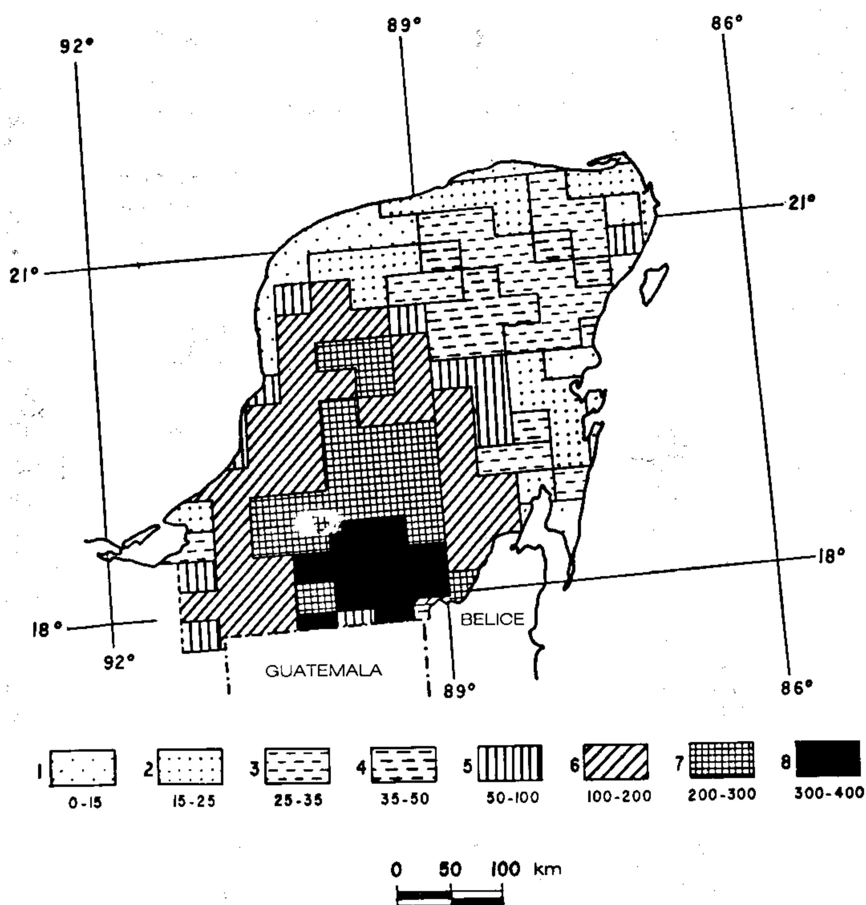
Figura 6.- Mapa de alturas máximas—valores en m s.n.m.m.
