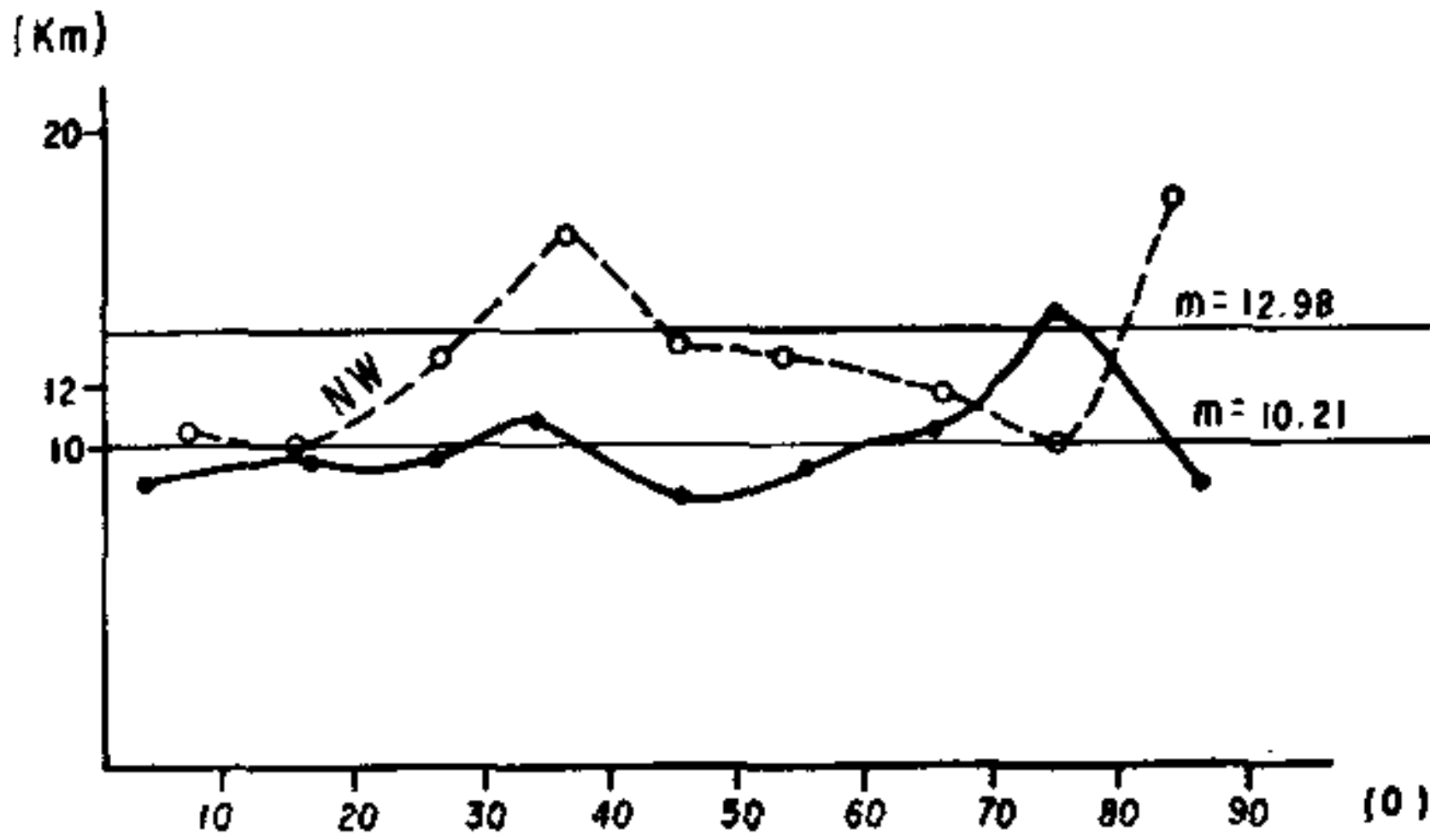
Figura 8.- Distribución gráfica de las longitudes de los lineamientos en los rangos de máxima concentración mostrados en la Figura 6.
