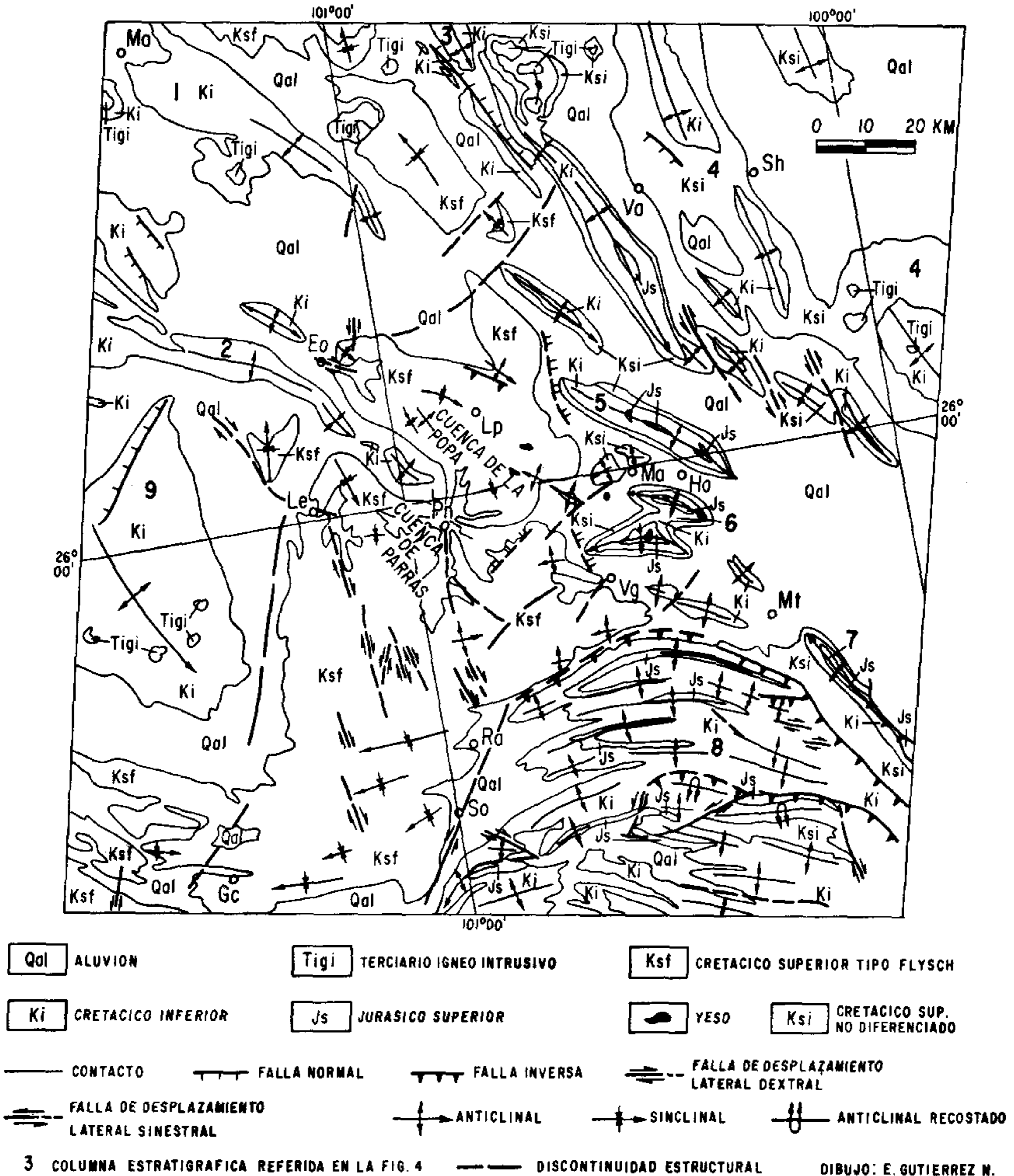
Figura 12.- Interpretación geológica de la imagen de satélite.
