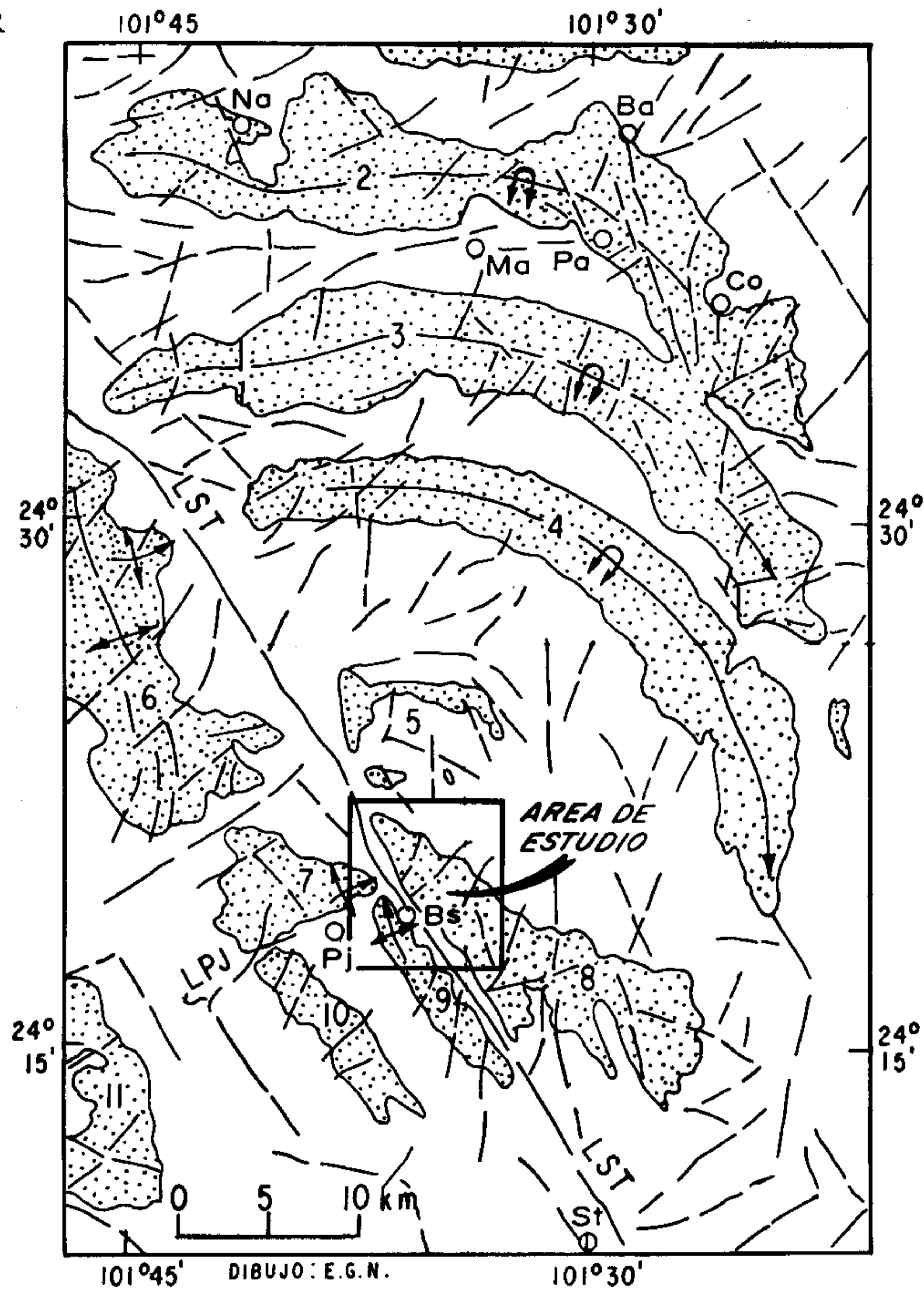
Figura 2.- Ubicación del área de estudio en el contexto regional, mostrando los lineamientos principales observados en la imagen de satélite y las sierras más importantes (áreas punteadas): 1. Sierra de Canutillo, 2. Sierra de la Caja. 3. Sierra de Santa Rosa, 4. Sierra Santa Rita, 5. Sierra de Tanquecillos, 6. Sierra de la Candelaria, 7. Sierra de las Iglesias, 8. Sierra de la Centella, 9. Sierra de los Escritorios, 10. Sierra del Barroso, 11. La Sierrita; Na, Nochebuena; Ba, Bonanza; Ma, Mazapil; Pa, Providencia; Co, Concepción del Oro; Pj, Presa del Junco; Bs, Banderitas; St, San Tiburcio; LST, Lineamiento de San Tiburcio; LPJ, Lineamiento de la Presa del Junco. El área enmarcada corresponde a la superficie cubierta por la Figura 4.
