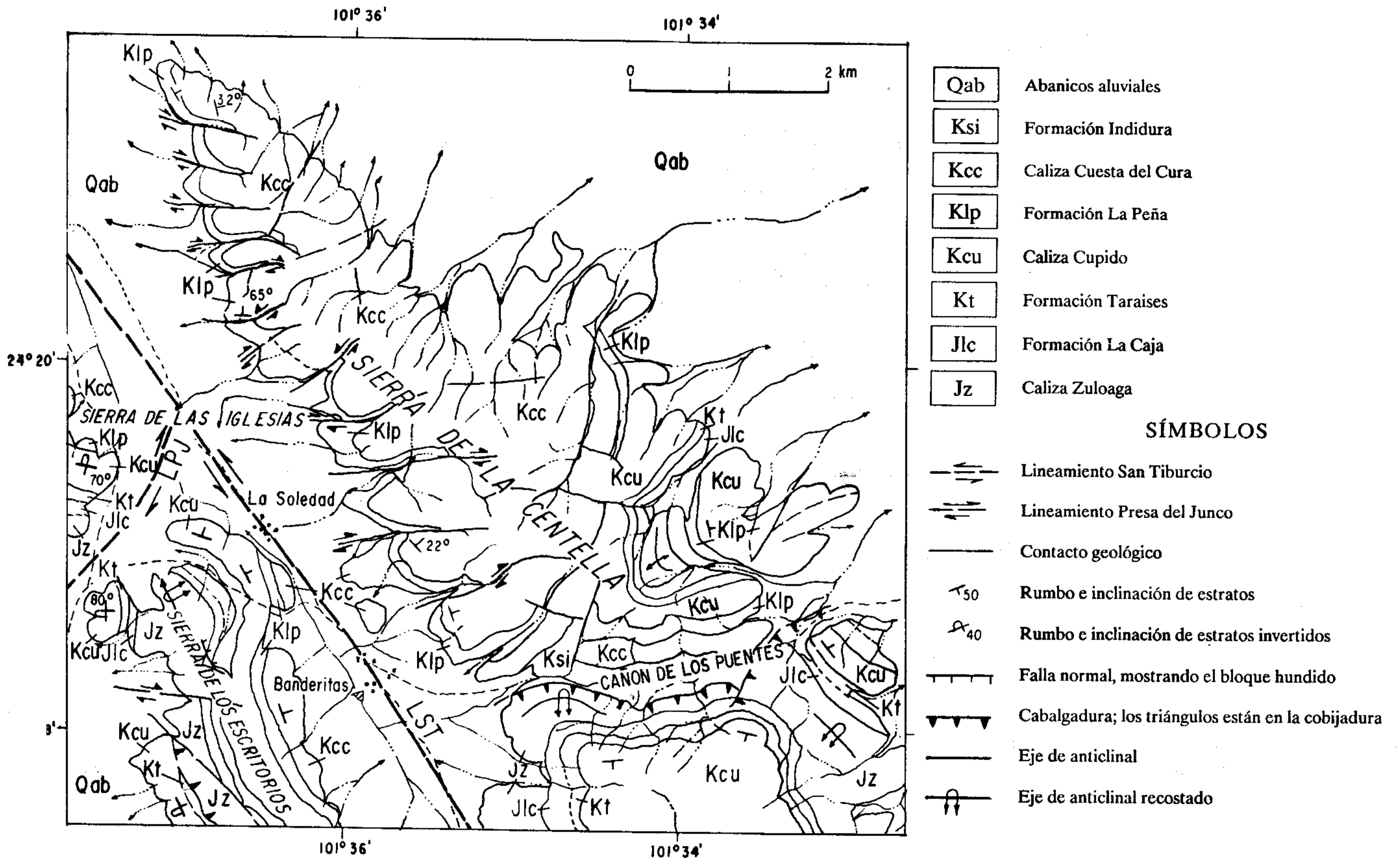
Figura 4.- Mapa geológico del área de estudio.
