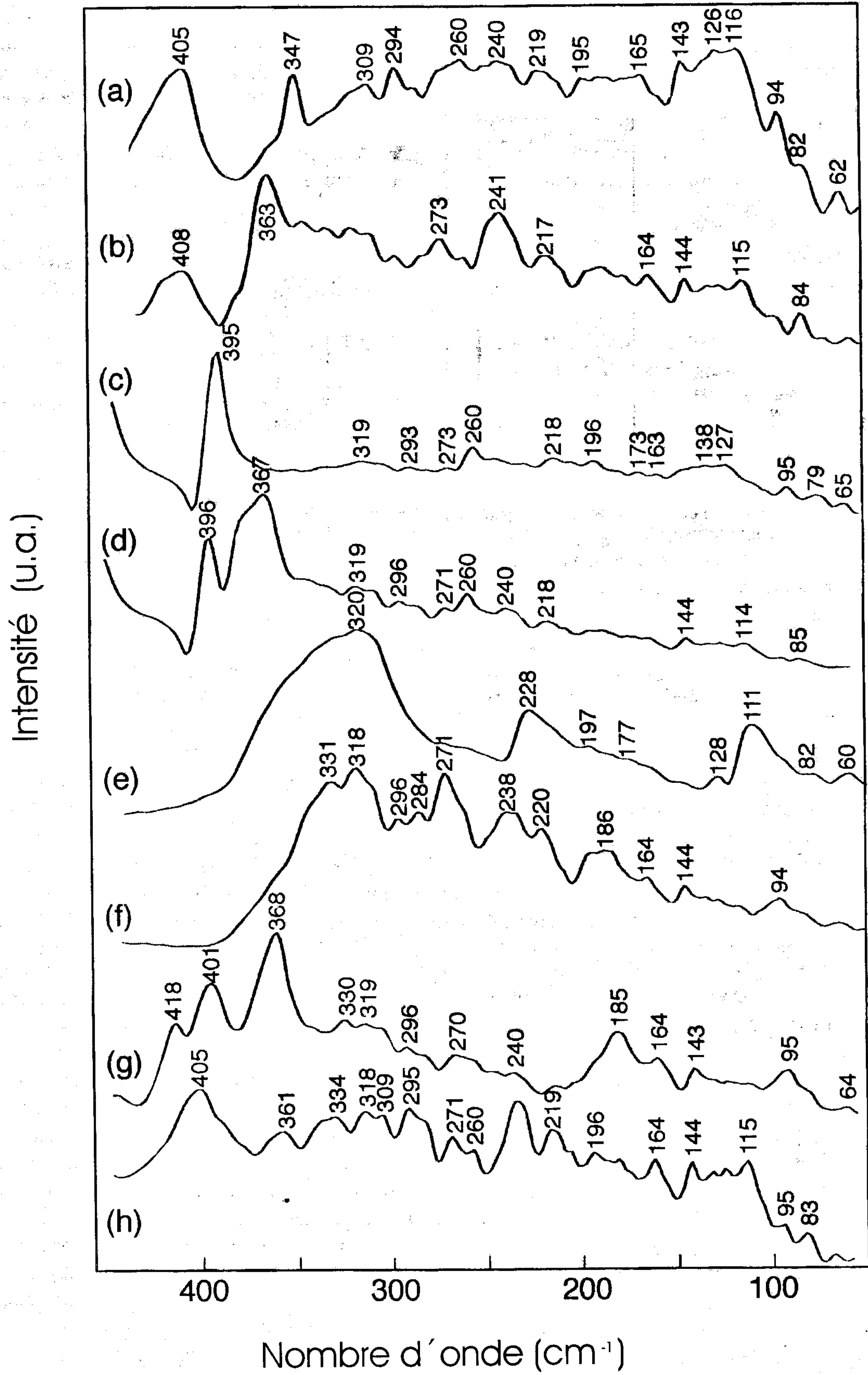
Figure 1: Spectres infrarouges de reflexion des mineraux dans le domaine lointain : A - Pyrite, B - Gibbsite, C - Quartz I c, D - Quartz II c, E - Calcite, F - Apatite, G - Oligoclase, H - Labradorite.
