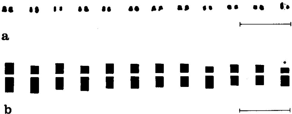
Fig. 3. a) Cariotipo de Karwinskia humboldtiana . Barra = 10 \mu m. b) Idiograma de K. humboldtiana . Barra= 3 \mu m. Para los tamaños cromosómicos absolutos e índice centromérico (véase cuadro 1).
